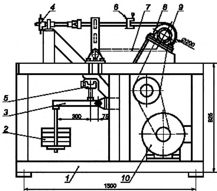
1 — станина; 2 — груз; 3 — рычаг; 4 — штурвал; 5 — нижний зажим; 6 — верхний зажим; 7 — образец ленты (сбегающая ветвь); 8 — образец ленты (набегающая ветвь); 9 — барабан; 10 — привод
