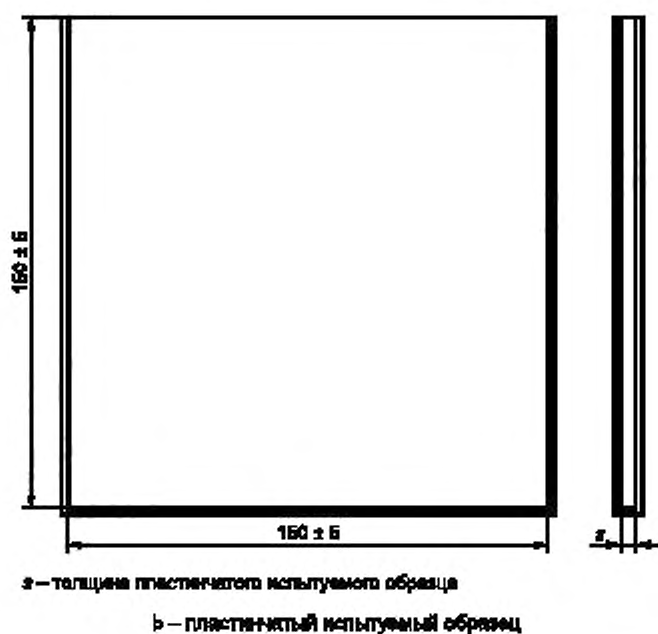
Рисунок 4 — Испытуемые образцы
