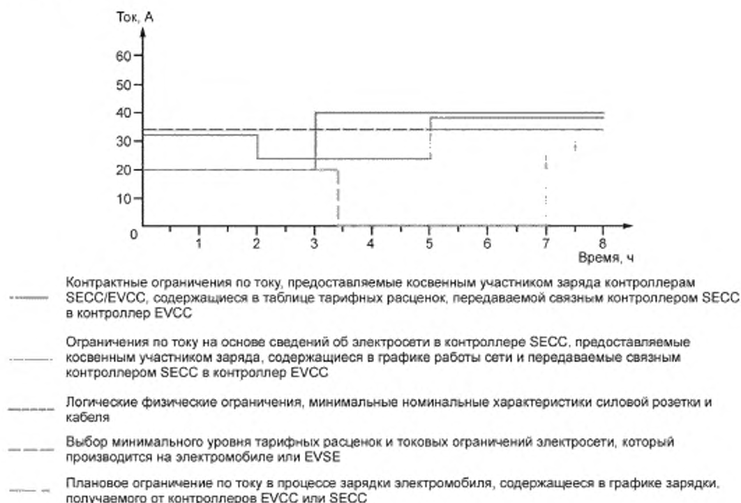
Рисунок А.5 — Эффекты планирования передаваемого тока
