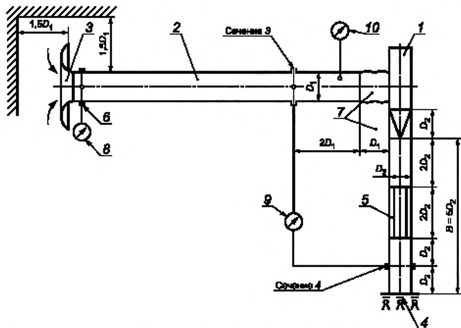
1 — испытуемый вентилятор; 2 — измерительный трубопровод; 3 — расходомер (сопло Вентури); 4 — дросселирующее устройство; 5 — струеуспокоитель; 6 — измерительное сечение в расходомере; 7 — переходные участки для присоединения вентилятора к измерительным воздухопроводам; 8 — устройство для измерения разности давлений в расходомере; 9 — устройство для измерения разности статических давлений до и после вентилятора; 10 — термометр для измерения температуры в трубопроводе
