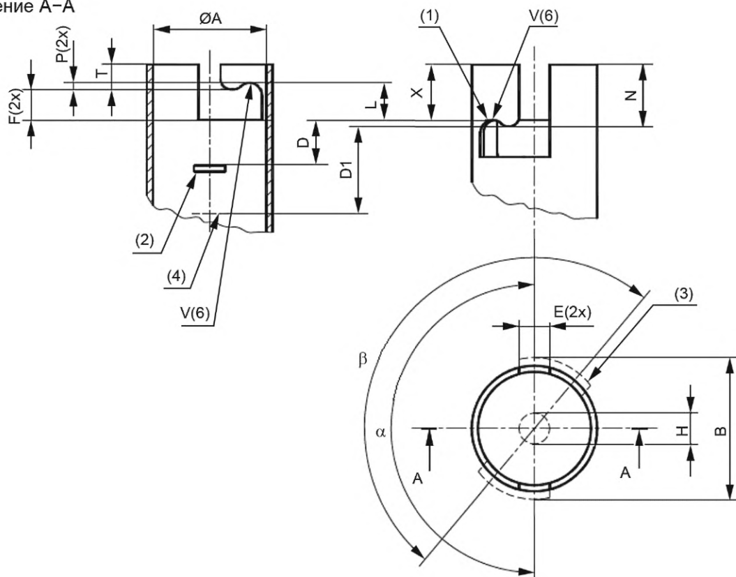
Сечение А-А
