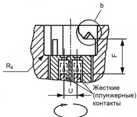
Сечение III-III
