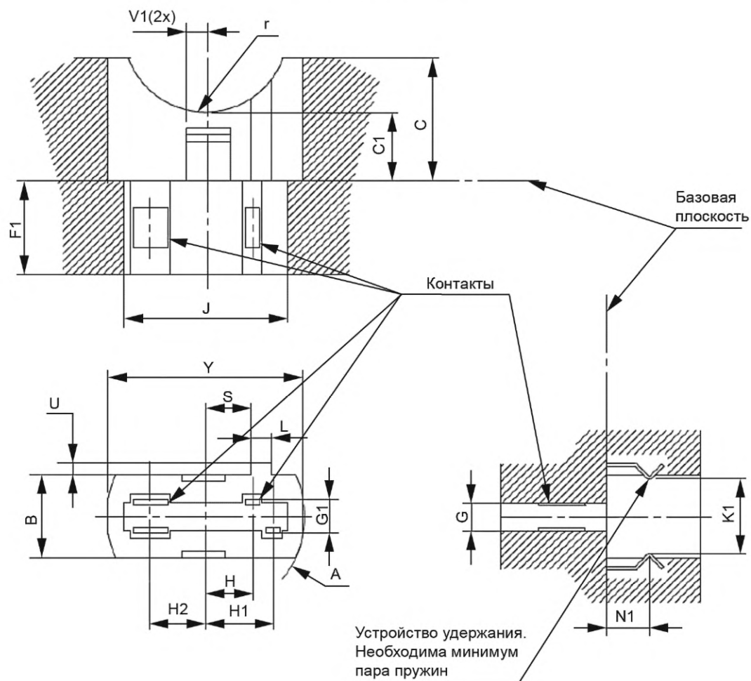
Форма базового паза
