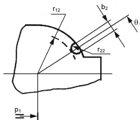
Сечение II-II
