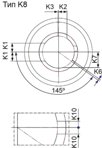
Деталь В (типы К4, К5, К6)
