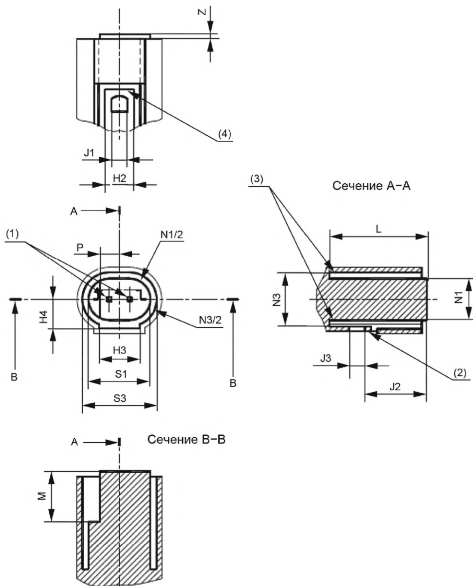
Соединитель PU20d
