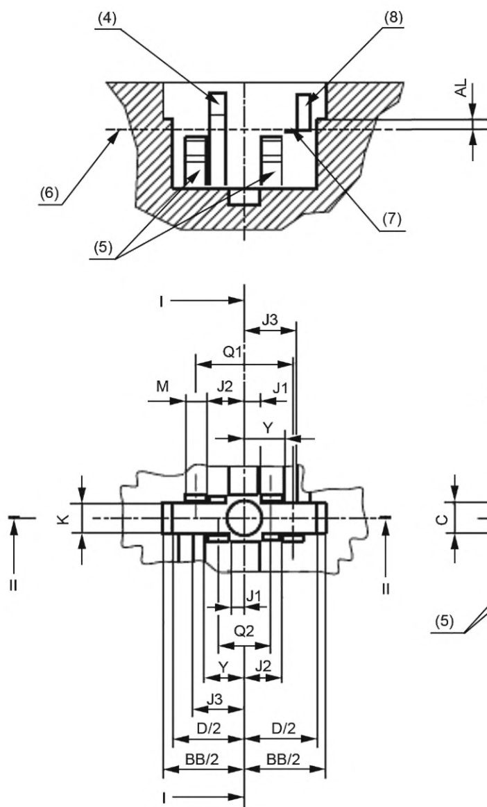
Сечение II-II
