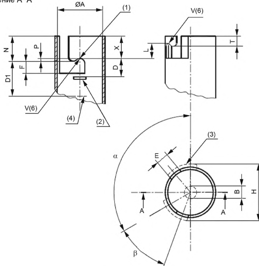
Сечение A-A
