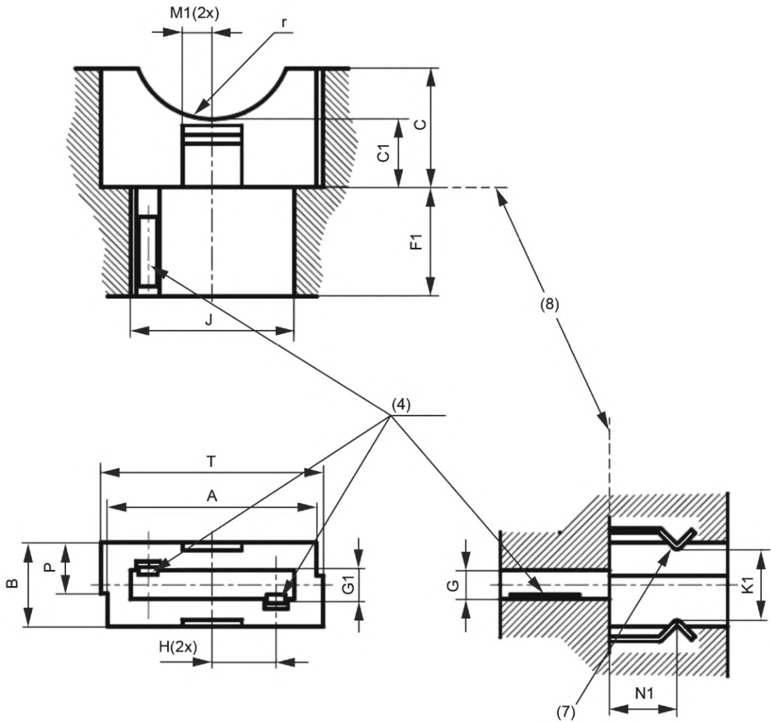
Патрон типа А
