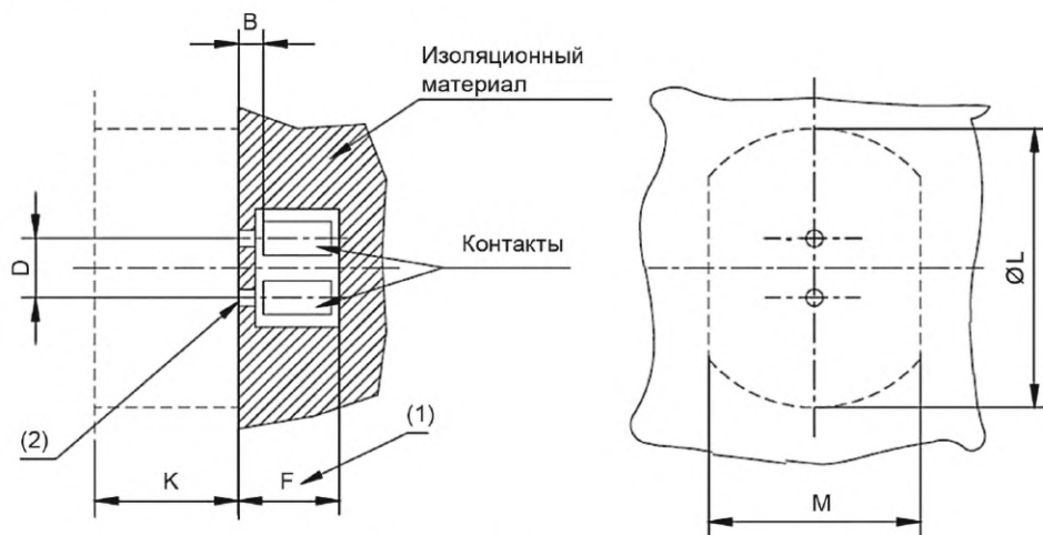
Рисунок 1 — Соединитель
