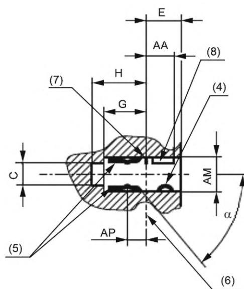
Сечение I-I
