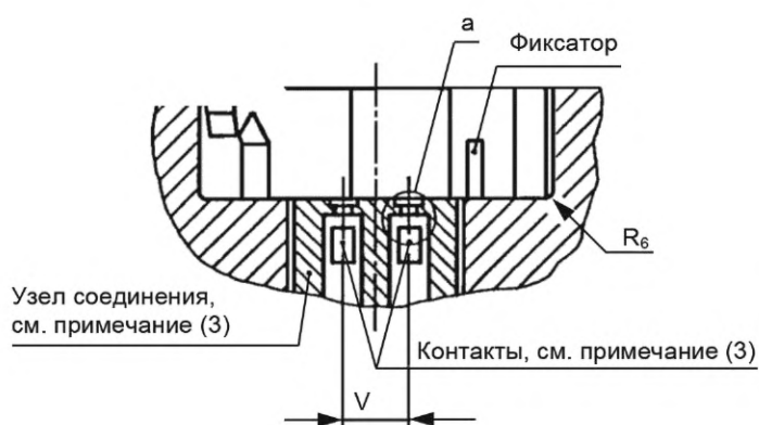
Сечение I-I
