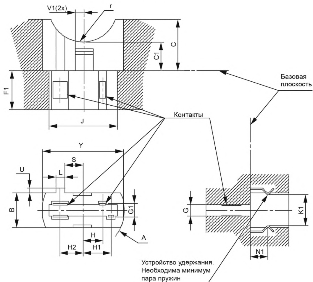
Форма базового паза
