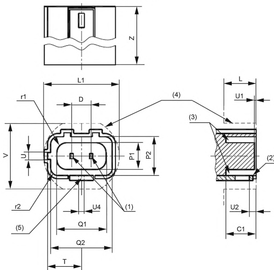
Соединитель PG20
