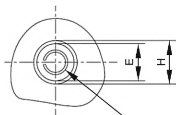
Осевое вставление
