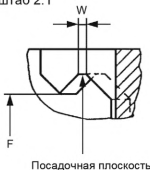
Деталь b Масштаб 2:1
