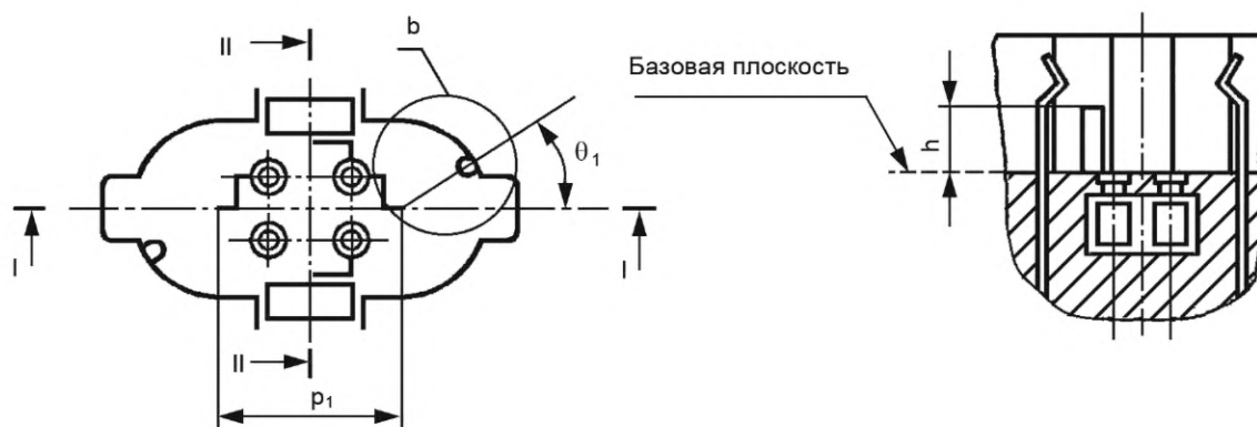
Сечение II-II
