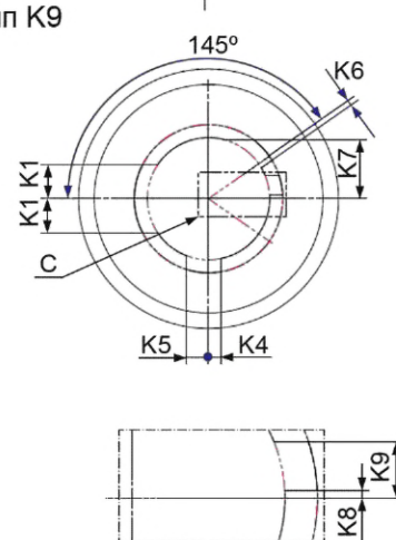
Деталь С (типы К7, К8, К9)
