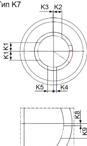
Деталь А (типы К1, К2, К3)
