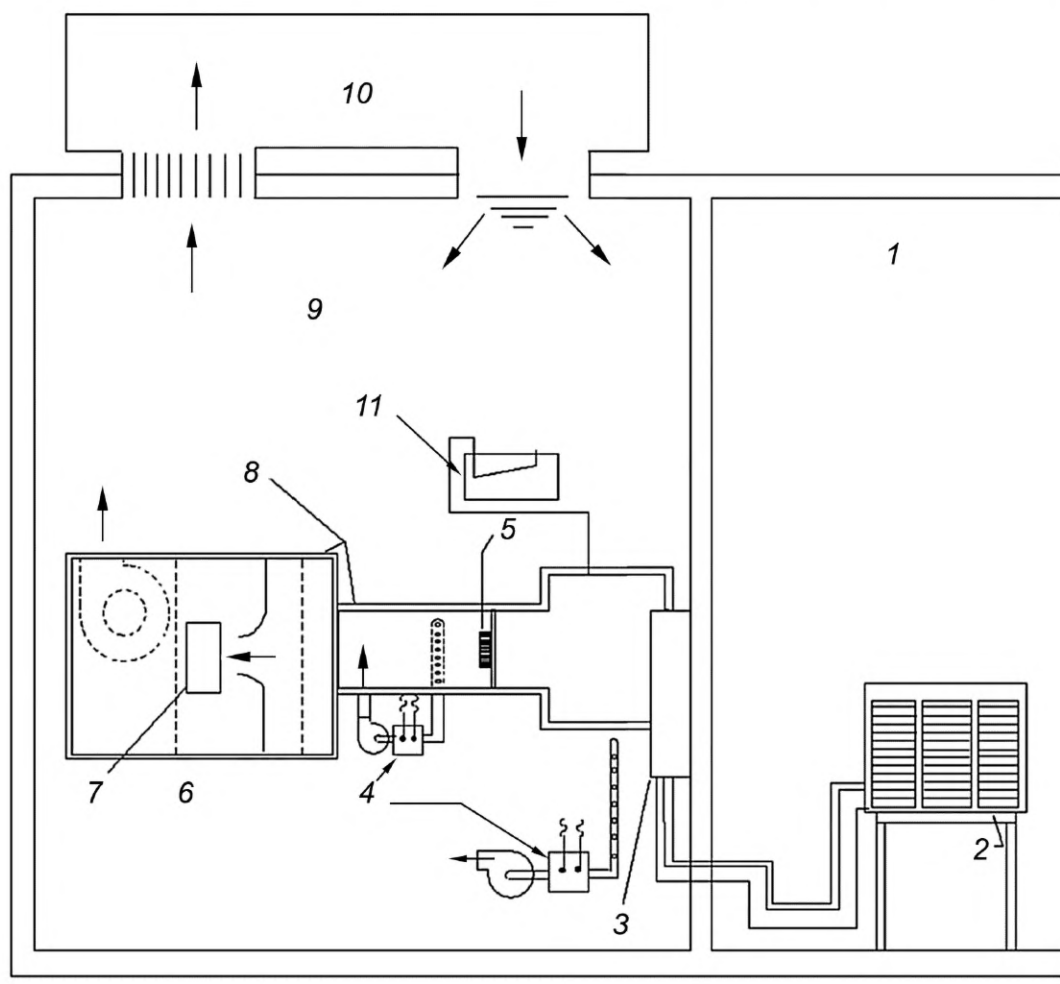
1 — отсеки наружной стороны; 2 — наружный блок испытываемого оборудования; 3 — секция испытываемого оборудования с внутренним теплообменником; 4 — измерительные приборы температуры и влажности; 5 — смеситель; 6 — аппарат измерения воздушного потока; 7 — дверь/окно; 8 — изоляция; 9 — отсеки внутренней стороны; 10 — аппарат кондиционирования помещения; 11 — аппаратура для измерения перепада давления
