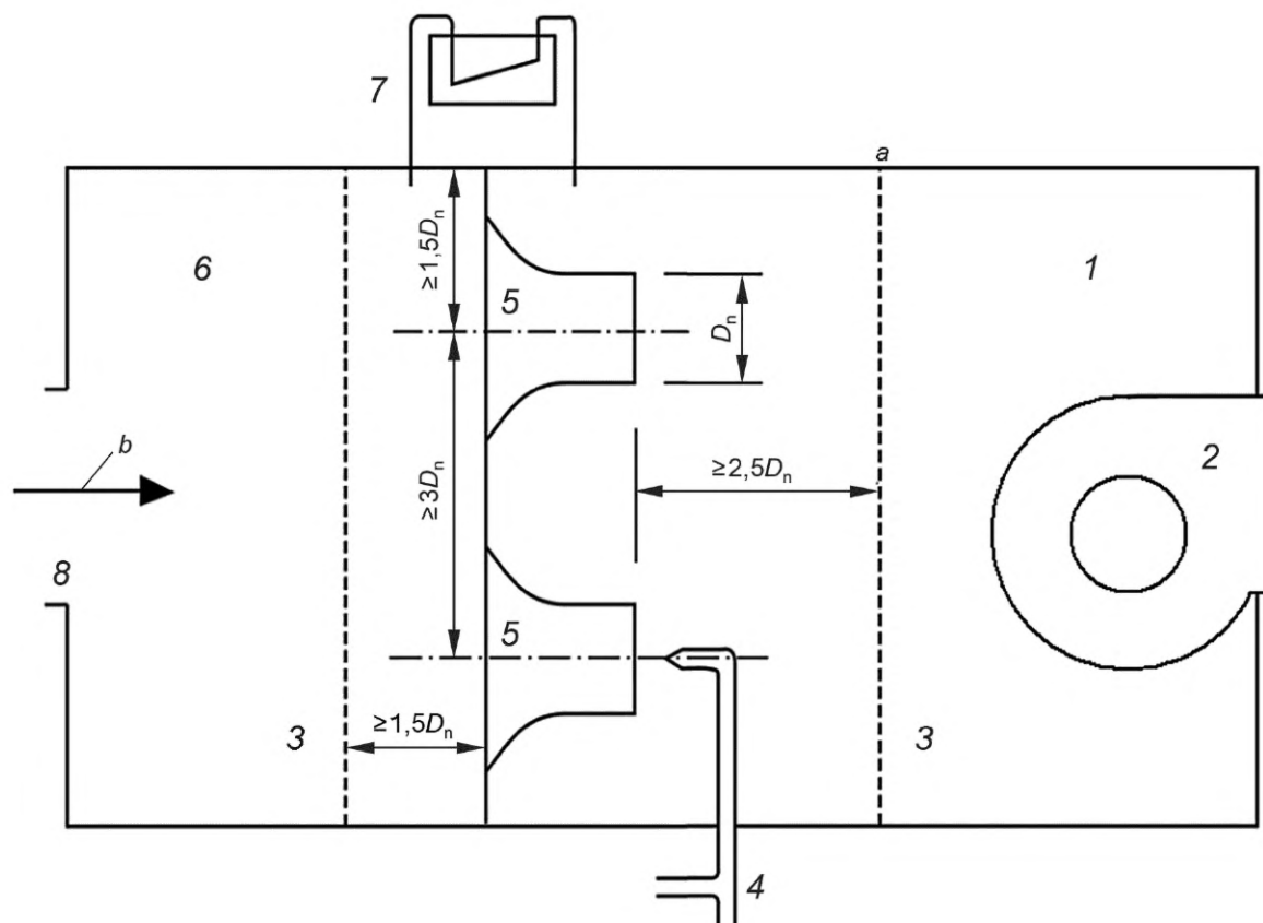
1 — разгрузочная камера; 2 — вытяжной вентилятор; 3 — рассеивающая перегородка; 4 — трубка Пито; 5 — сопло; 6 — приемная камера; 7 — аппаратура измерения дифференциального давления; 8 — воздуховод-переходник (см. С.5.1); D_n — диаметр горловины сопла; а — рассеивающие перегородки (следует перфорировать, сохраняя приблизительно 40 % свободного пространства); b — воздушный поток
