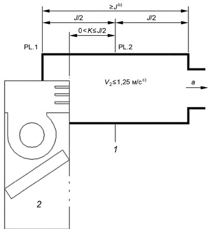
a — направление к отборнику воздуха и аппарату измерения воздушного потока; b) J = 2D_e , где D_e = \sqrt{4AB/\pi} ; A и B — размеры выпускных отверстий оборудования; c) V_2 — средняя скорость воздуха 1 — наконечники в отверстиях измерения статического давления; 2 — исследуемое оборудование
