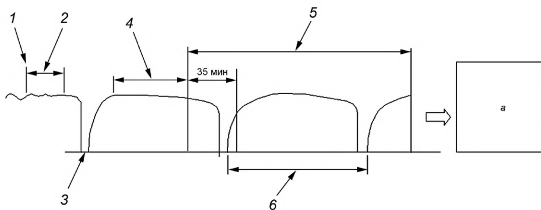
Рисунок Q.4 — Испытание теплопроизводительности с одним циклом размораживания в течение периода сбора данных
