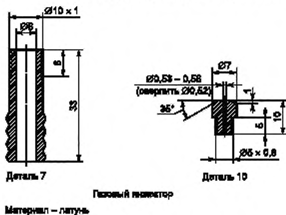
Рисунок А.4 — Детали горелки (3)
