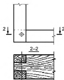
Рисунок Б.2 — Каркас с элементами сплошного сечения
