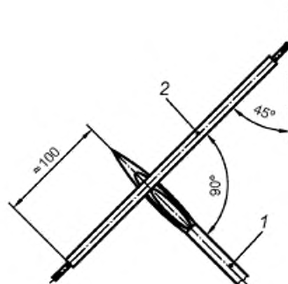
1 — горелка Бунзена; 2 — образец
