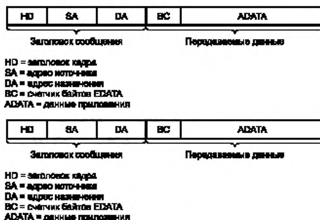
Рисунок 5 — Кадр обычного сообщения
