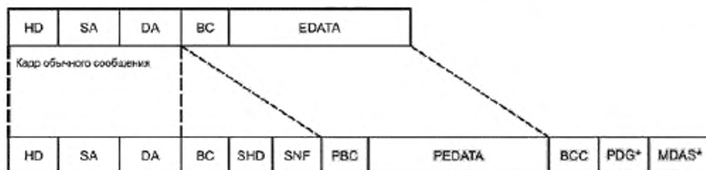
Рисунок 6 — Кадр защищенного сообщения
