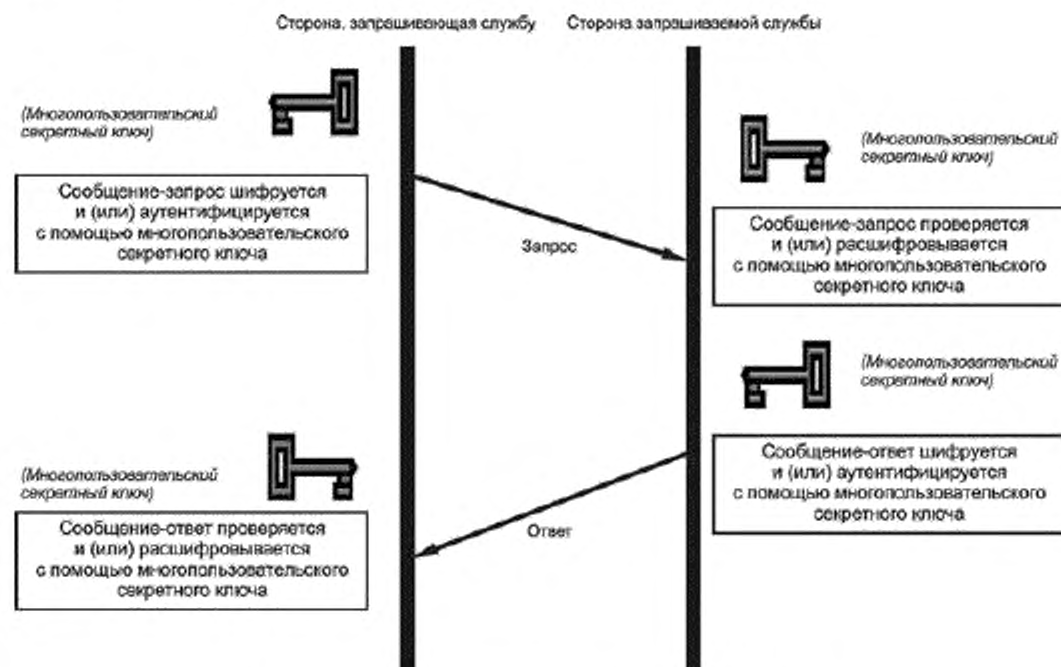
Рисунок 3 — Взаимодействие сторон на основе протокола SCPM
