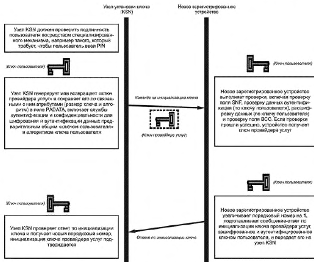
Рисунок 17 — Последовательности инициализации ключа провайдера услуг
