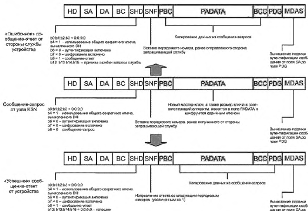
Рисунок 21 — Кадры защищенного сообщения по обновлению мастер-ключа. Обмен ключом с использованием общего секретного ключа DH
