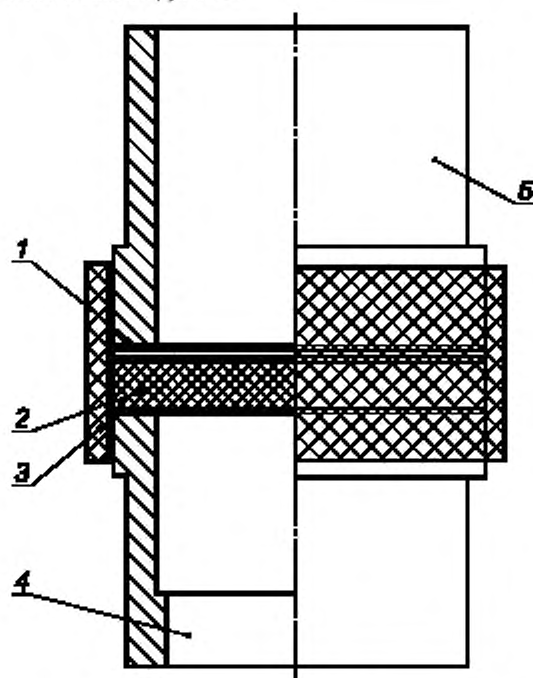
Рисунок 1 — Устройство для фильтрации (левая половина показана в разрезе)
