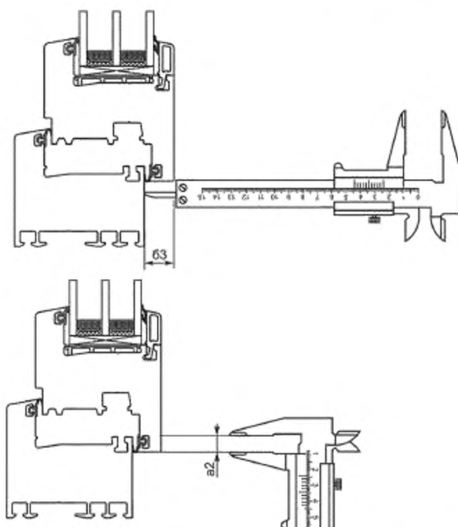
Рисунок Г.6 — Определение величины рабочего напlava створки
