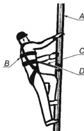
A — жесткая анкерная линия; B — страховочная привязь; C — шнор, D — устройство ползункового типа
