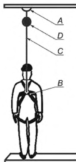
A — анкерная точка, B — страховочная привязь; C — втягивающийся шнор (отдельная деталь средства защиты втягивающего типа); D — страховочное устройство (средство защиты втягивающего типа)
