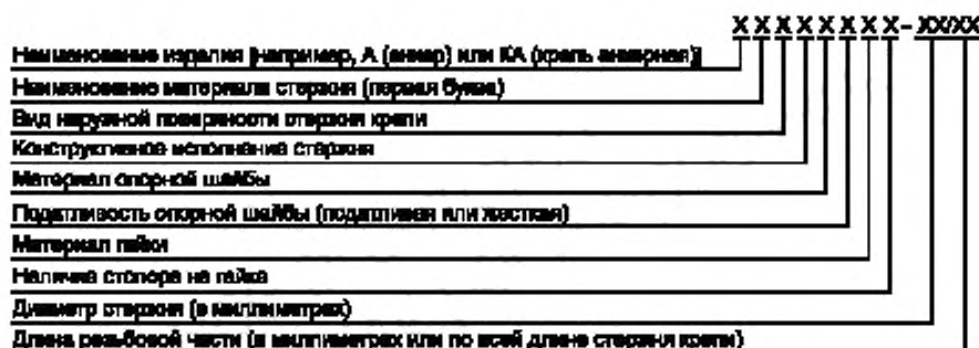
Рисунок 2 — Пример формирования обозначения крепежа
