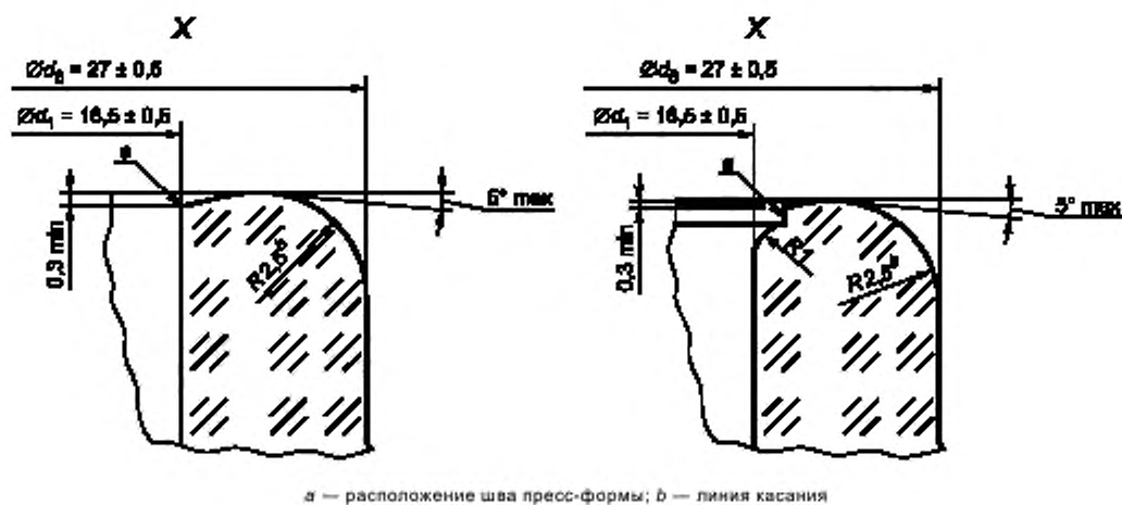
Рисунок 2 — Деталь горловины X
