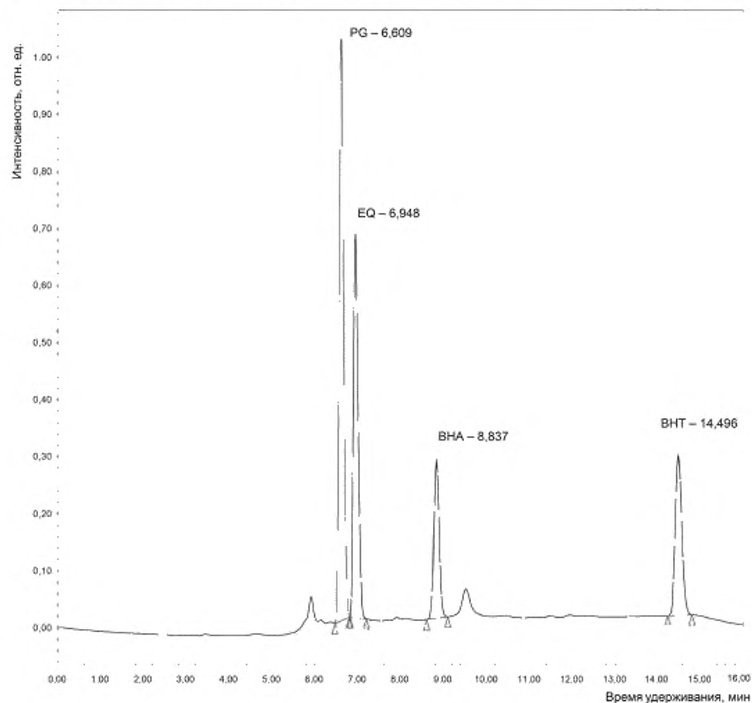
Рисунок А.2 — Хроматограмма градуировочного раствора антиоксидантов с массовой концентрацией 0,1 \text{ мг/см}^3 , полученная на колонке 1 (см. А.1)
