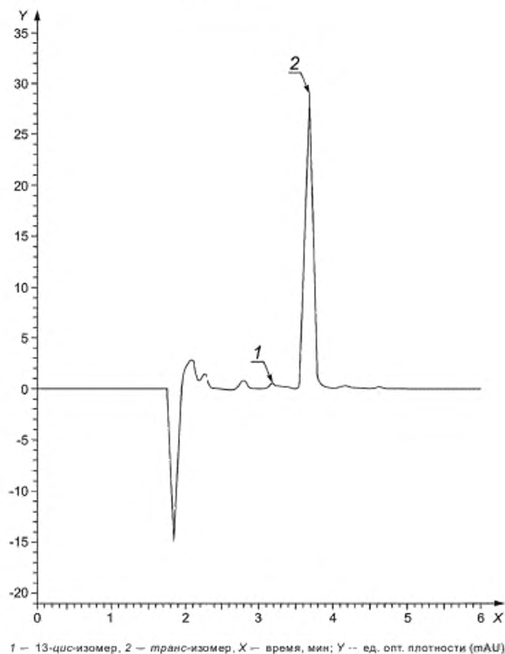
1 — 13-цис-изомер, 2 — транс-изомер, X — время, мин; Y — ед. опт. плотности (mAU) Рисунок А.1 — Хроматограмма градуировочного раствора ретинола пальмитата
