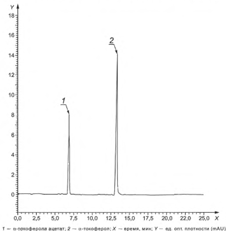
Рисунок А.5 — Хроматограмма градуировочного раствора смеси \alpha -токоферола ацетата и \alpha -токоферола
