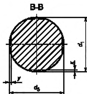
Рисунок 10 — Сплюсывание участков, поперечное сечение В-В на рисунке 9
