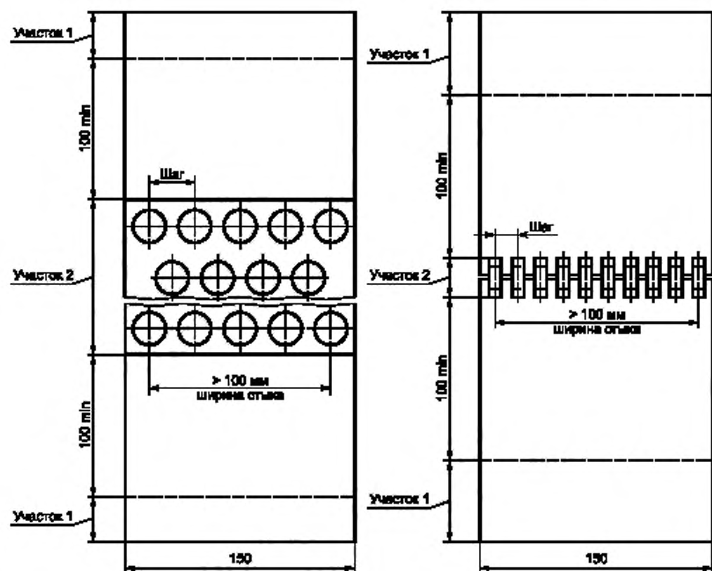
Рисунок 1 — Образцы неразъемного механического соединения
