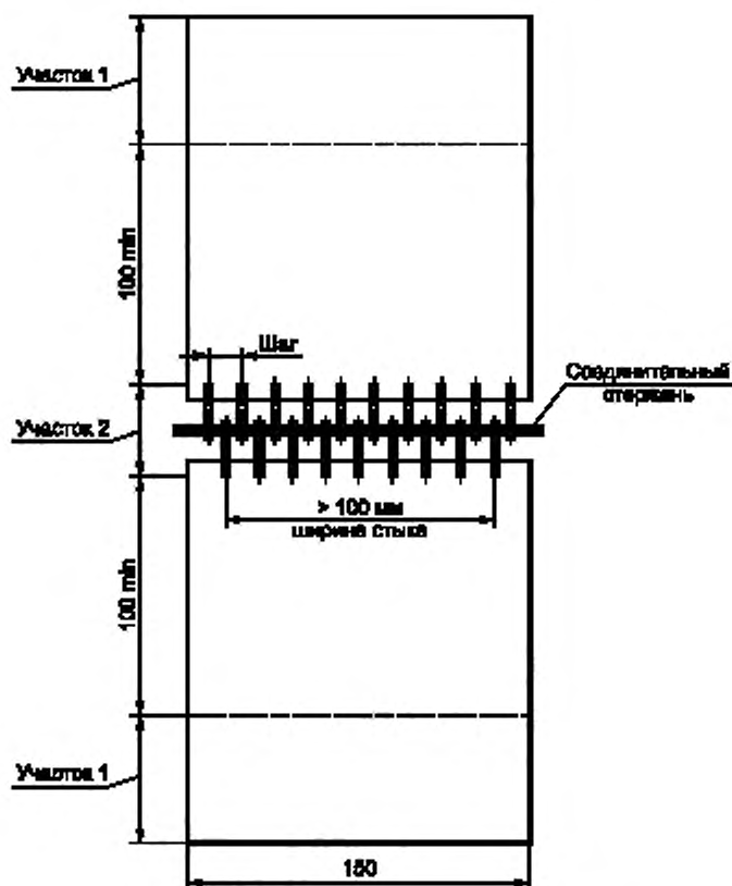
Рисунок 2 — Образец разъемного механического соединения
