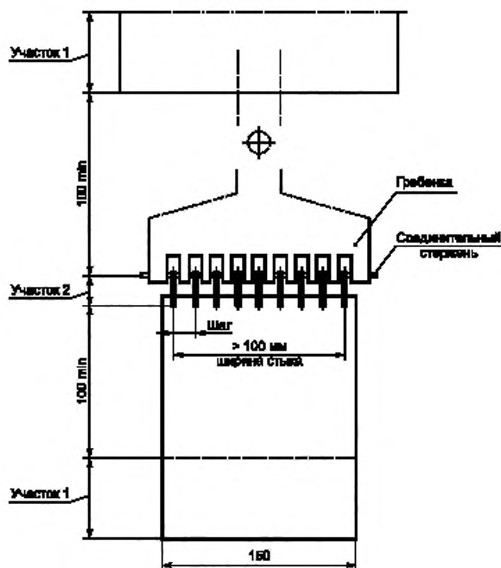
участок 1 — участок зажима ленты; участок 2 — механический стык
