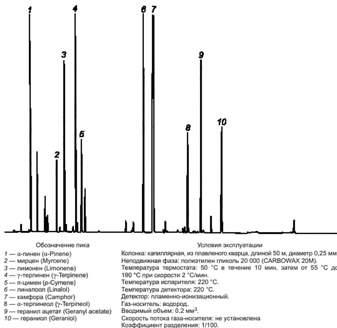
Рисунок А.2 — Типичная хроматограмма, полученная на полярной колонке
