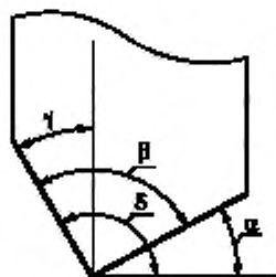
Рисунок 1 — Конструктивные углы
