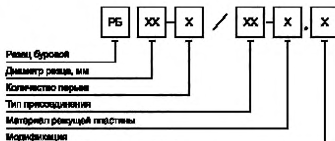
Рисунок 3 — Схема условного обозначения
