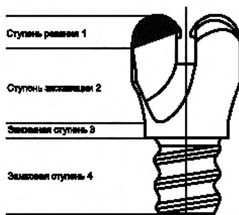
Рисунок 2 — Конструкция бурового резца
