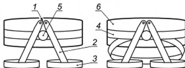
1 — точка крепления (состоящая из двух элементов крепления); 2 — лямки, соединяющие петли, охватывающие ноги, с поясным привязным ремнем; 3 — петли, охватывающие ноги; 4 — поясной привязной ремень; 5 — элемент застегивания и регулировки; 6 — спинная опора
