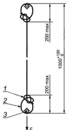
F — испытательный груз массой (100 \pm 1) кг или эквивалентная сила; 1 — узел булинь, 2 — петля заделки на конце; 3 — точка крепления
