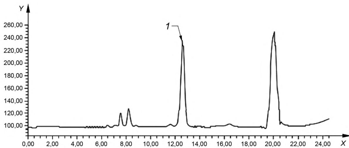
Рисунок А.1 — Типичная хроматограмма стандартного раствора
