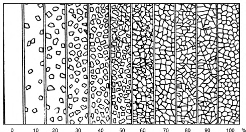
Рисунок 1 — Шкала сплоченности льда
