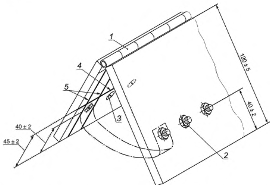
1 — петля; 2 — крепежная гайка; 3 — болт с потайной головкой; 4 — линия, параллельная шарниру для определения местоположения образцов для испытаний (только для метода с клейкой лентой); 5 — вспомогательная линия для определения местоположения образцов для испытаний (только для метода с клейкой лентой)
