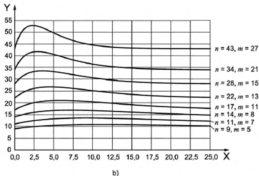
Рисунок 11 — Кривые среднего объема выборки для планов контроля числа несоответствий, неусеченный контроль с \alpha \leq 5\% и \beta \leq 10\%
