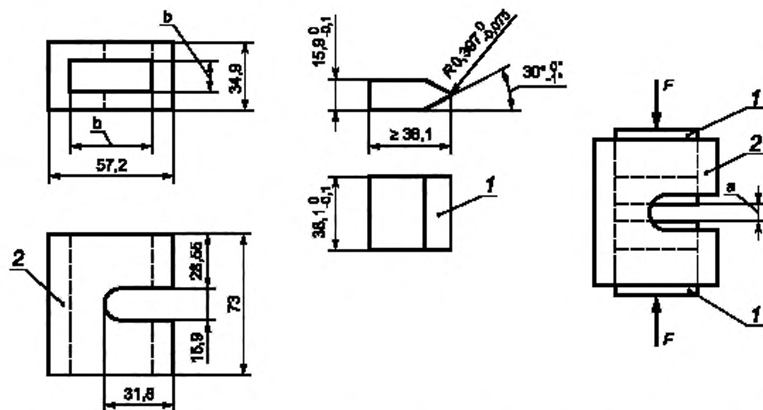
1 — режущие лезвия, механически обработанные из резцов с твердостью 60 HRC по шкале Роквелла; 2 — приспособление для испытаний на срез (соответствующие размеры зависят от окончательного размера заточенных режущих лезвий); F — прикладываемое срезающее усилие; a — 15,9 мм (5/8 дюйма), зазор реза для размещения ПУ во время испытания, b — на 0,1 мм больше, чем окончательная длина/ширина заточенного лезвия
