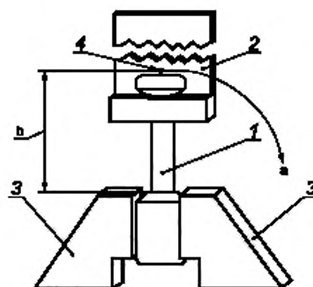
Рисунок 7 — Схема испытаний усиленных и защитных пломб стержневого типа на изгиб
