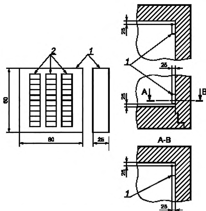
1 — монтажная пластинка; 2 — одноразовый термометр максимальных значений
