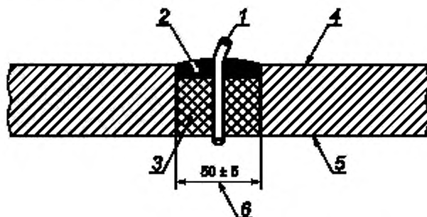
1 — кабельный ввод; 2 — силикон; 3 — минеральная вата, керамическое волокно или аналогичный материал; 4 — внутренняя сторона основания образца; 5 — наружная сторона основания образца; 6 — диаметр отверстия
