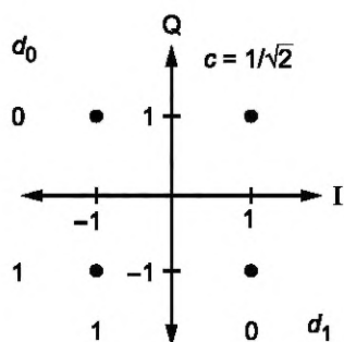
Рисунок 4 — Созвездие QPSK
