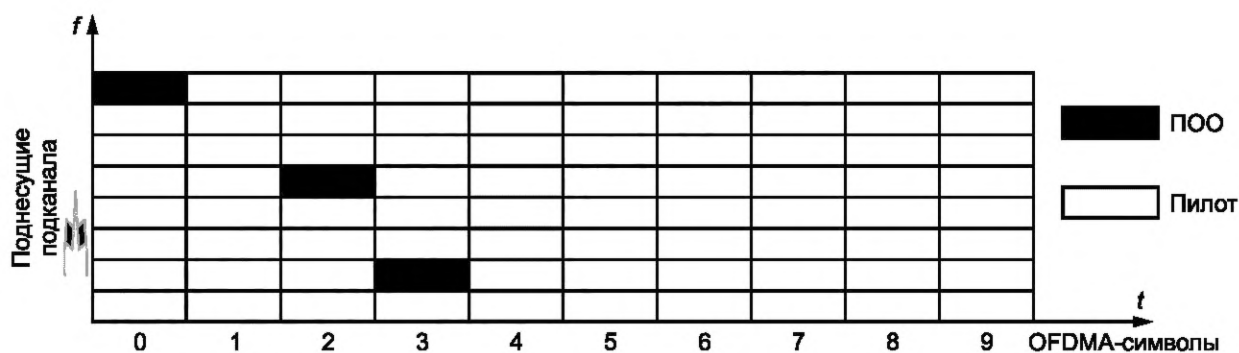
Рисунок 23 — Структура стационарного подканала (ПдК) для супер-тайм-слота
