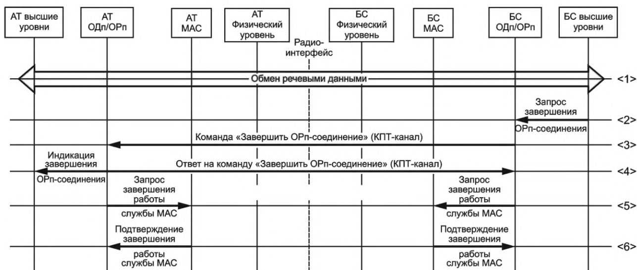
Рисунок 55 — Процедура «Завершение соединения ОРп-подуровня по инициативе БС»
