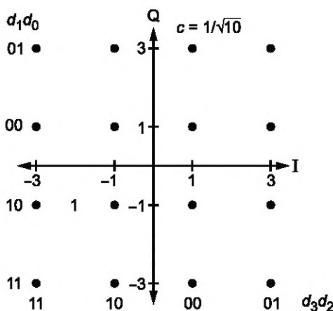
Рисунок 6 — Созвездие 16QAM
