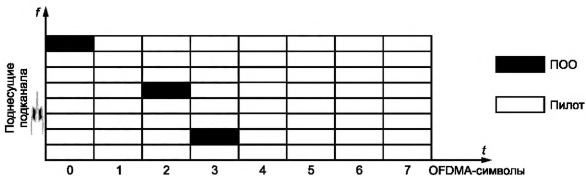
Рисунок 22 — Структура стационарного подканала (ПдК) для обычного тайм-слота
