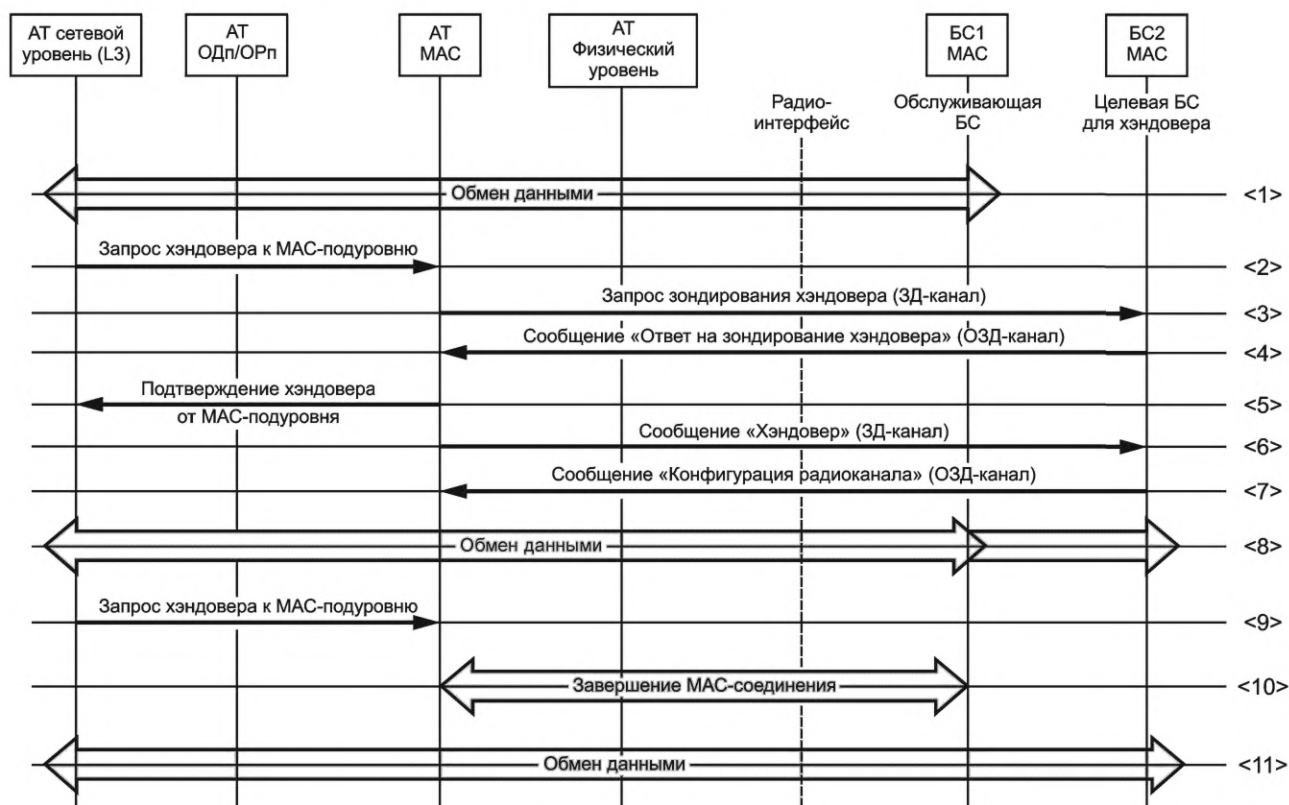
Рисунок 60 — Процедура «Хэндовер»
