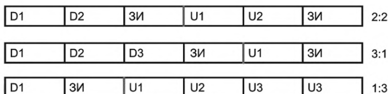
Рисунок 19 — Распределение тайм-слотов в радиолиниях DL/UL для кадра длительностью 5 мс
