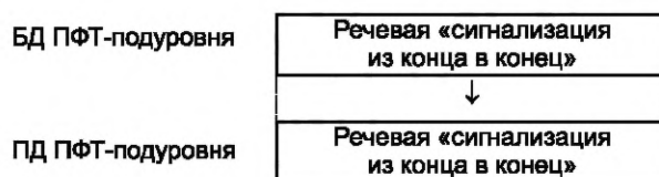
Рисунок 40 — Формирование ПД ПФТ из пакета речевой «сигнализации из конца в конец»
