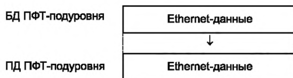
Рисунок 37 — Формирование ПД ПФТ-подуровня из Ethernet-данных (режим без шифрования)
