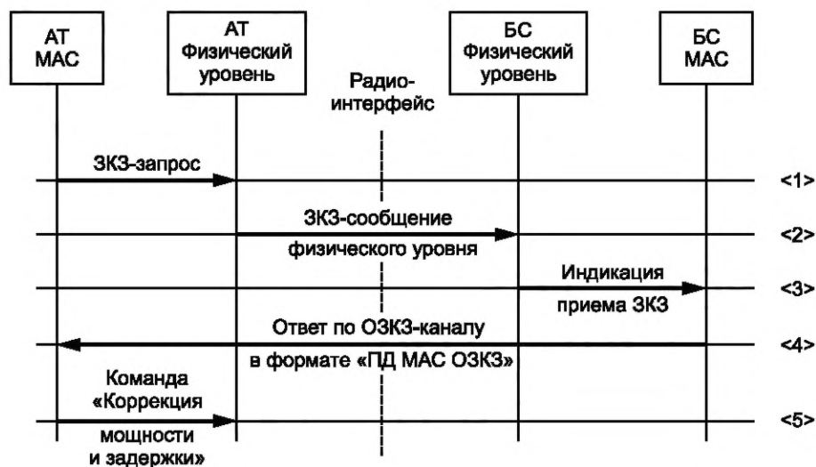
Рисунок 41 — ЗКЗ-процедура
