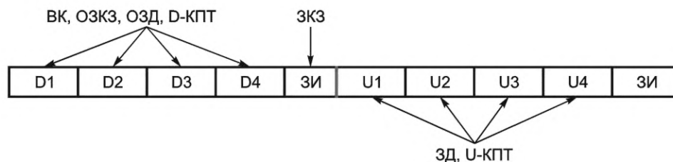
Рисунок 26 — Размещение физических каналов на временных интервалах кадра
