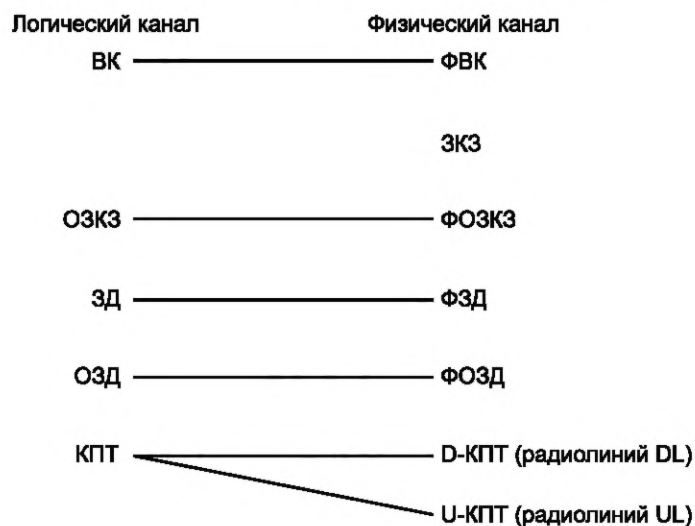
Рисунок 29 — Отображение логических каналов на физические каналы
