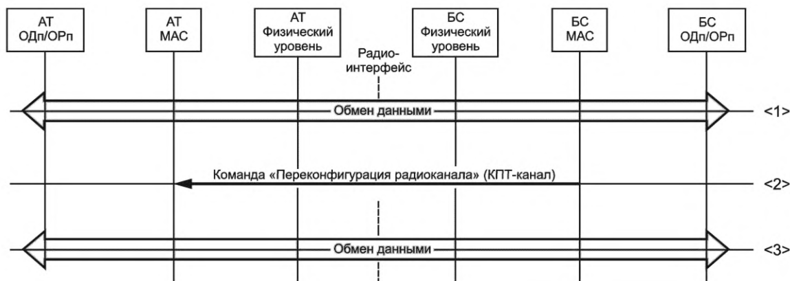
Рисунок 53 — Процедура «Переконфигурация (изменения полосы) радиоканала», осуществляемая БС
