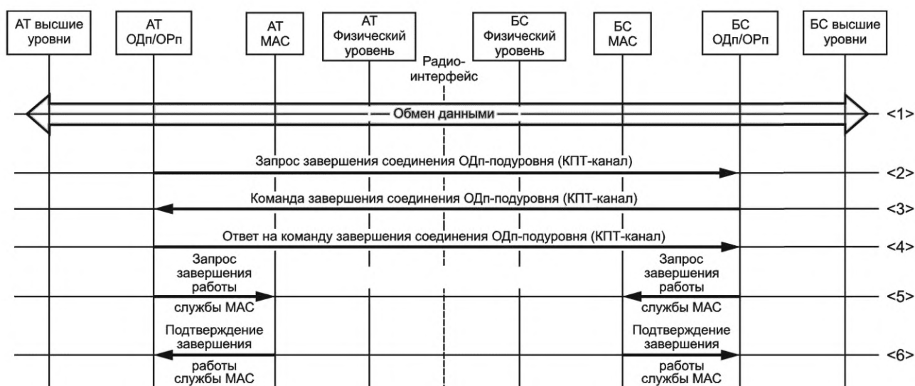
Рисунок 56 — Процедура «Завершение соединения ОДп-подуровня по инициативе АТ»
