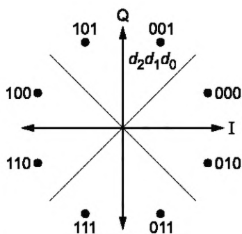
Рисунок 5 — Созвездие 8PSK
