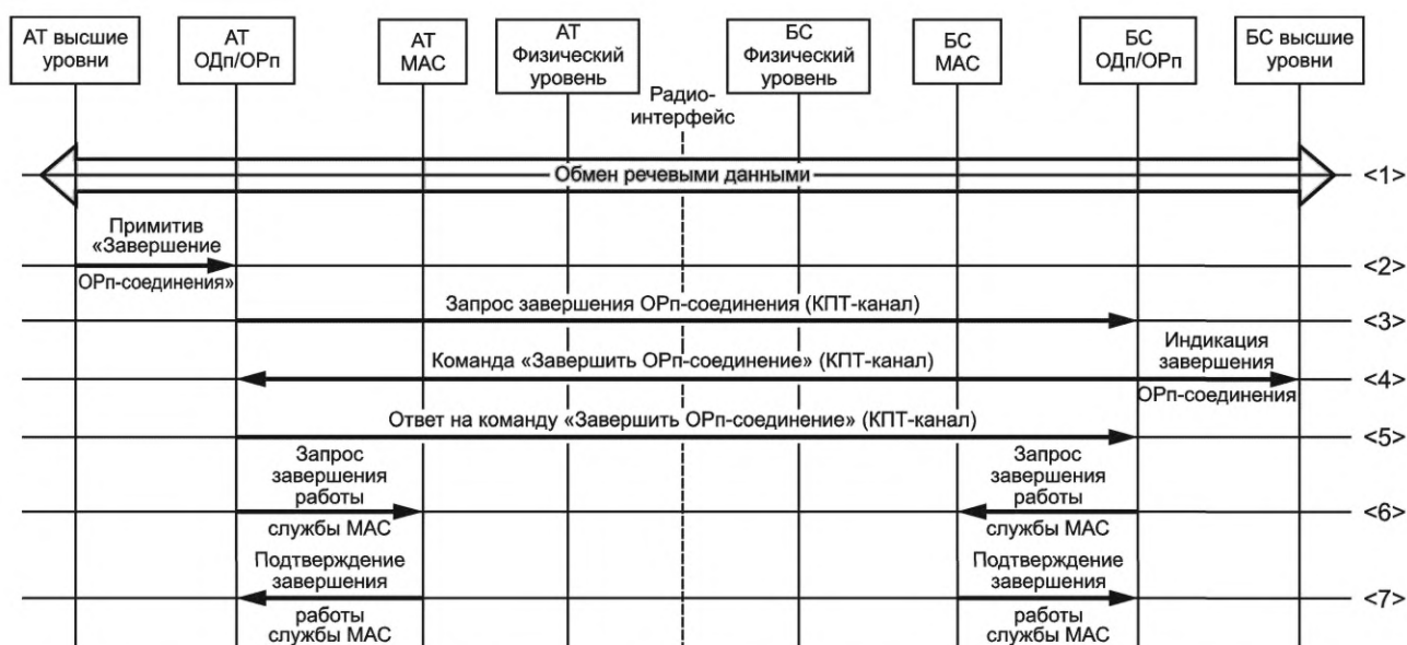
Рисунок 54 — Процедура «Завершение соединения ОРп-подуровня по инициативе АТ»
