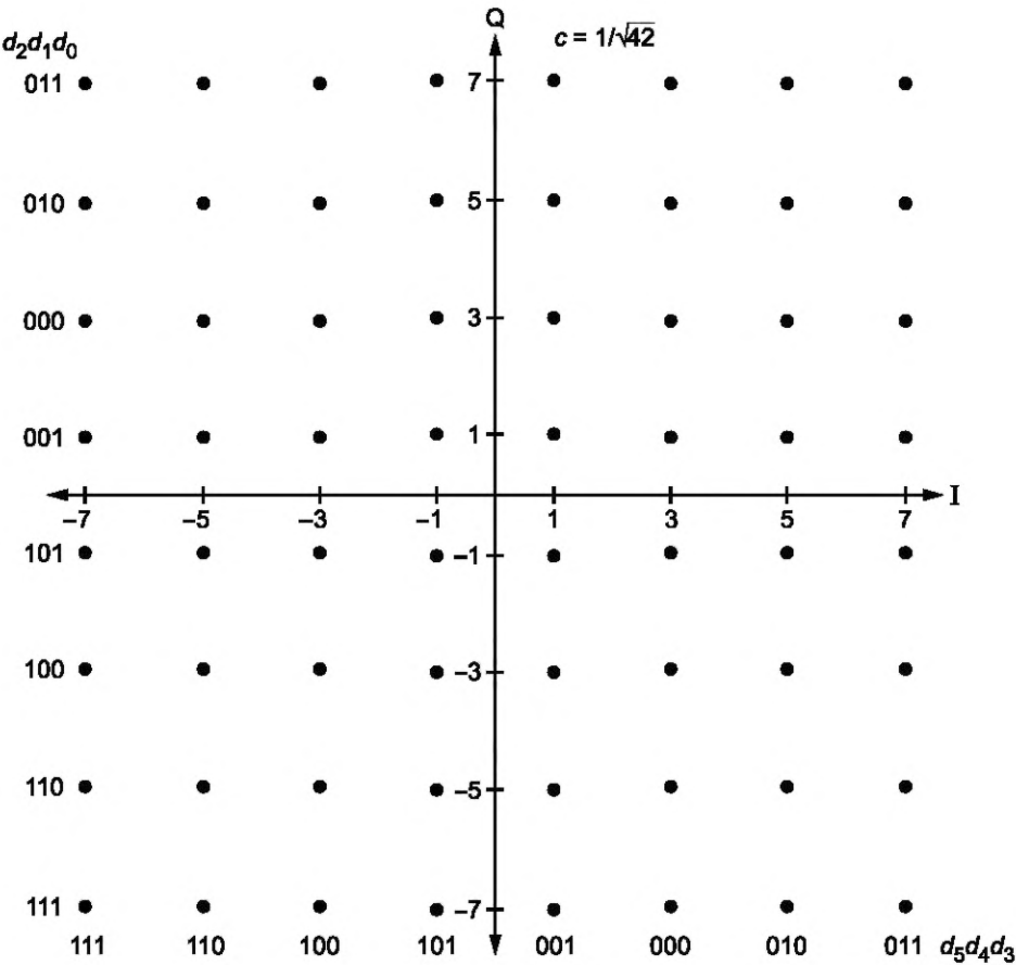
Рисунок 7 — Созвездие 64QAM
