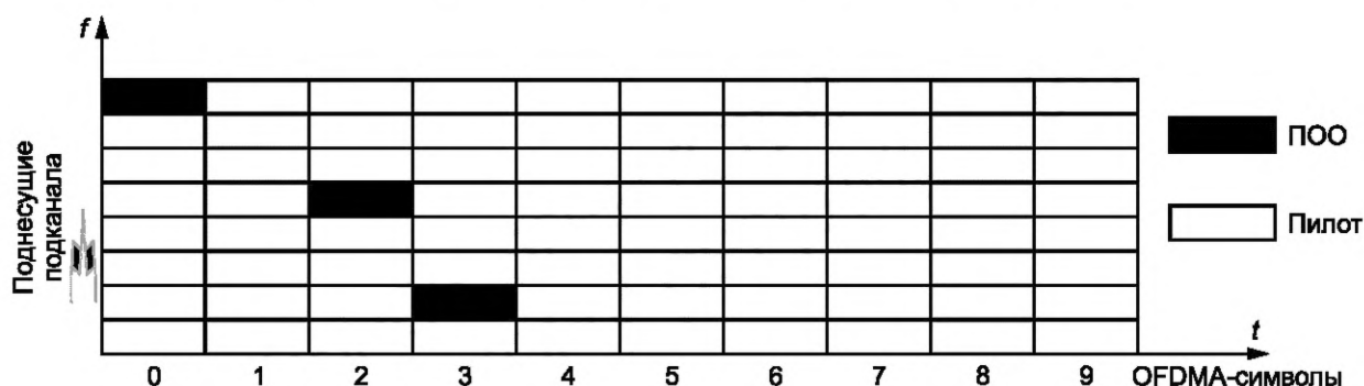
Рисунок 25 — Структура мобильного подканала (ПдК) для супер-тайм-слота
