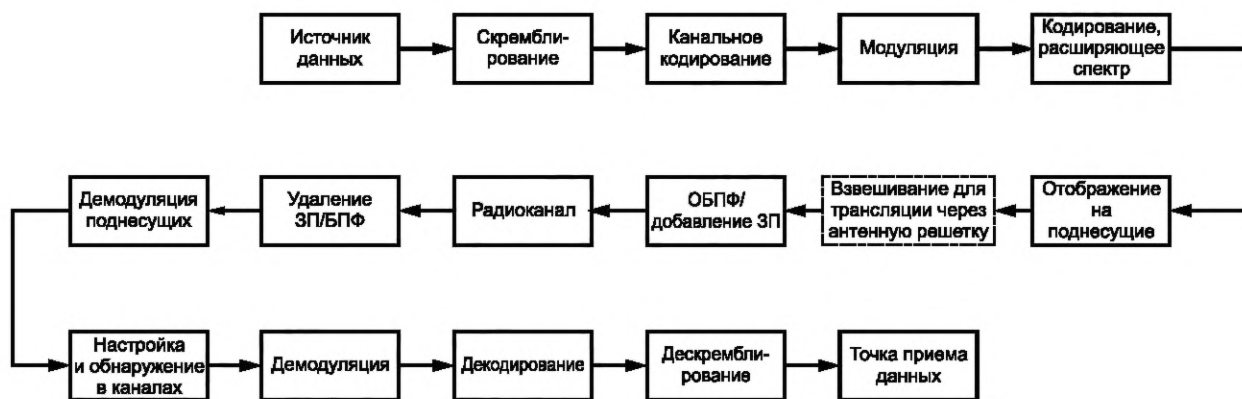
Рисунок 2 — Преобразование потока данных в радиолинии DL
