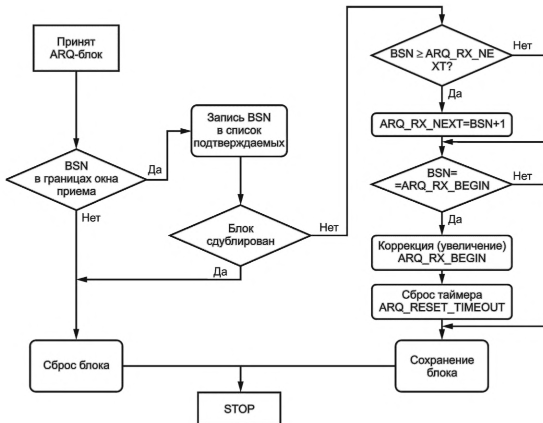
Рисунок 32 — Алгоритм работы в режиме ARQ
