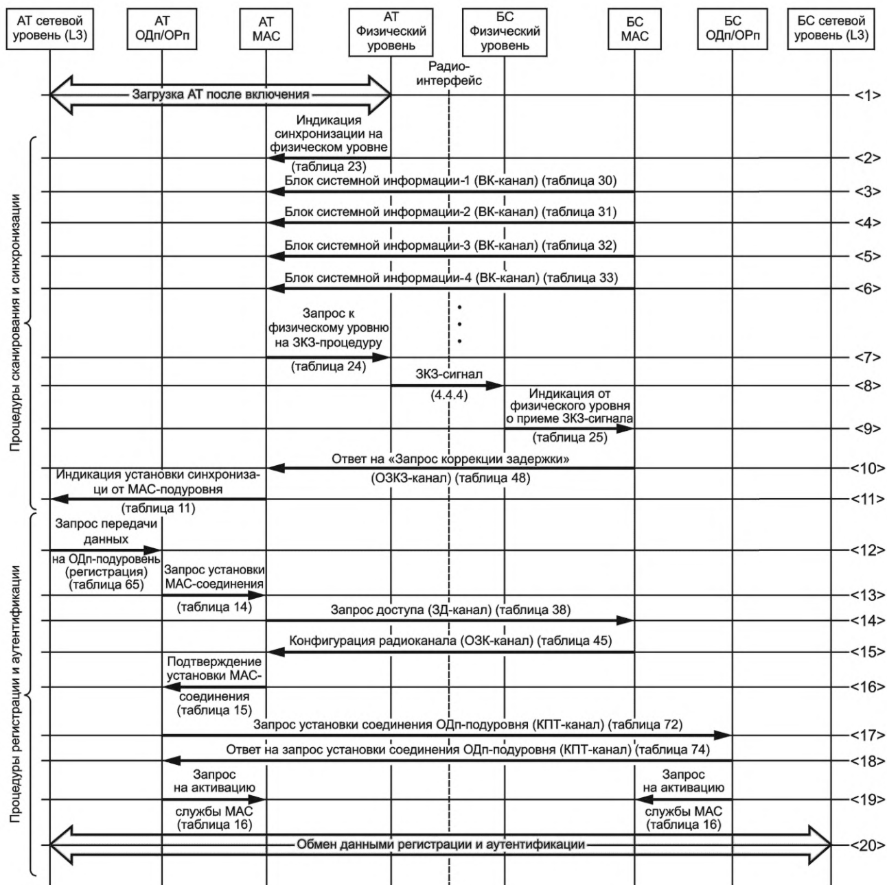
Рисунок 62 — Процедура «Доступ к сети и инициализация»
