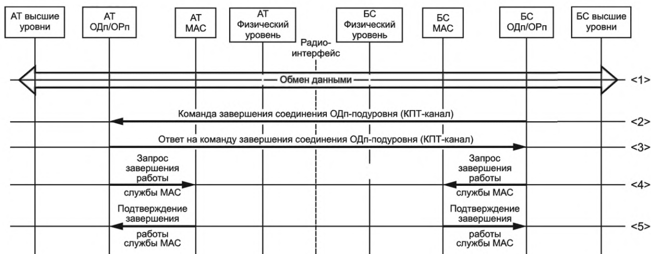
Рисунок 57 — Процедура «Завершение соединения ОДп-подуровня по инициативе БС»
