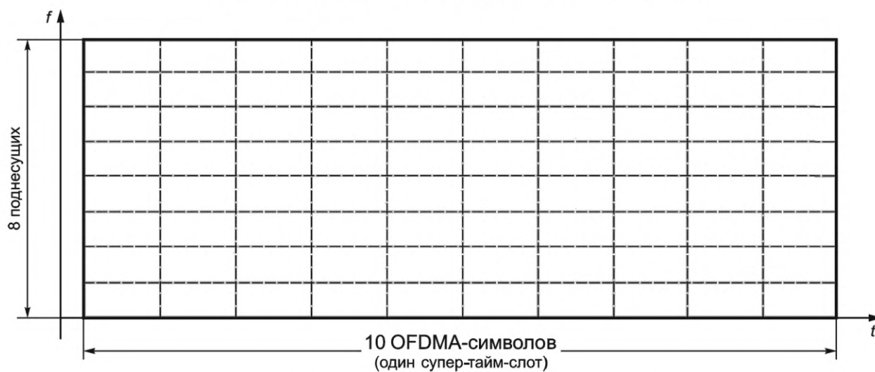
Рисунок 21 — Структура подканала (ПдК) в супер-тайм-слоте
