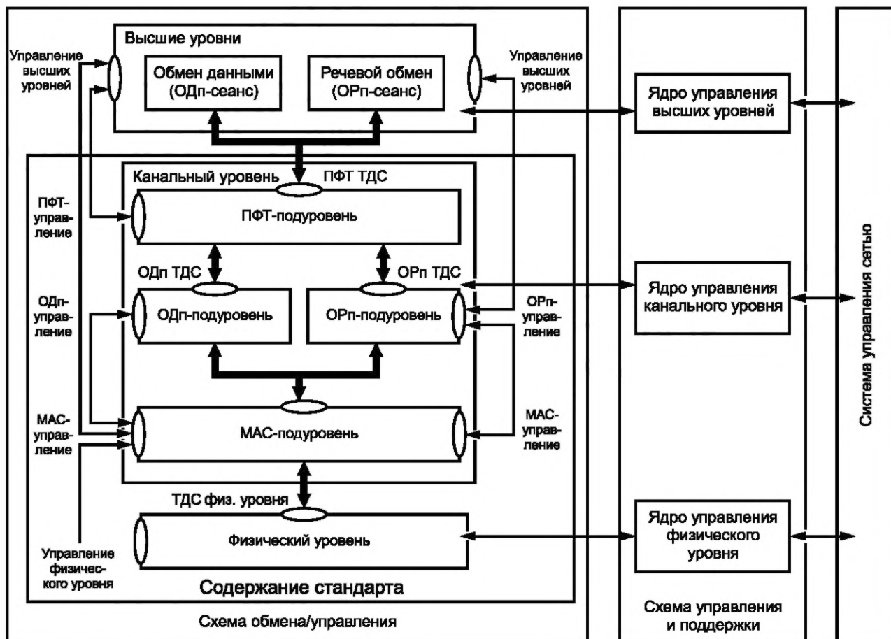
Рисунок 28 — Эталонная архитектура протоколов
