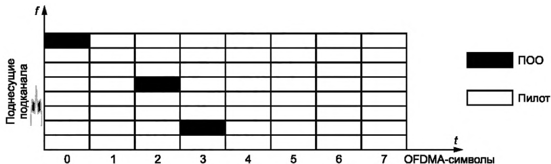
Рисунок 24 — Структура мобильного подканала (ПдК) для обычного тайм-слота
