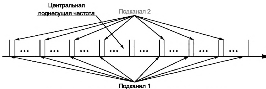
Рисунок 9 — Частотно-спектральная структура OFDMA-символа
