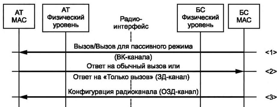
Рисунок 43 — Процедура «Вызов»
