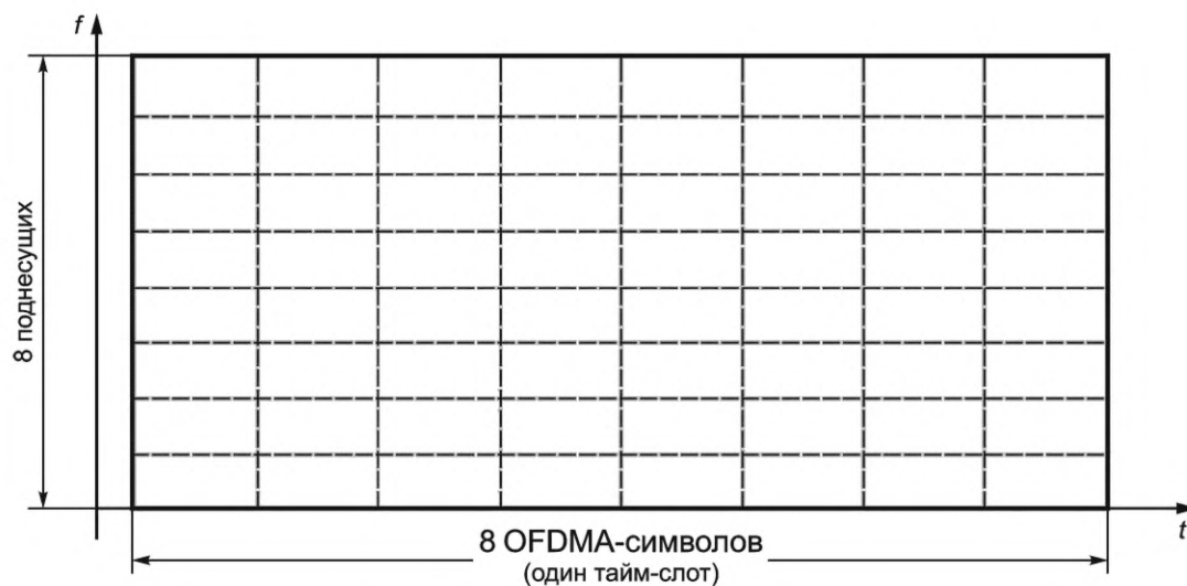
Рисунок 20 — Структура подканала (ПдК) в обычном тайм-слоте
