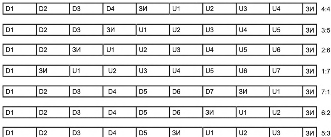
Рисунок 18 — Распределение тайм-слотов в радиолиниях DL/UL для кадра длительностью 10 мс
