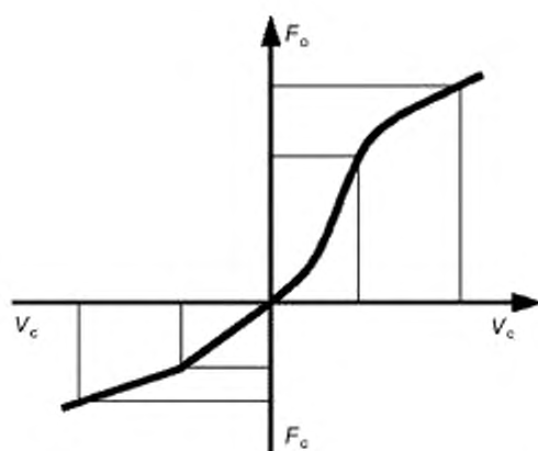
Рисунок 4 — Зависимость сопротивления амортизатора от скорости перемещения поршня
