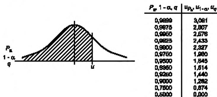
Рисунок 1 — Квантили стандартного нормального распределения
