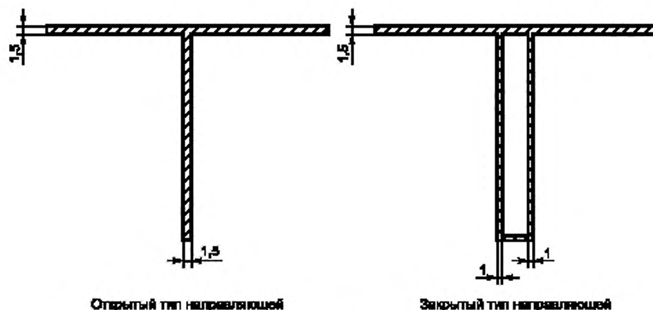
Рисунок 1 — Типы направляющих из алюминиевых сплавов
