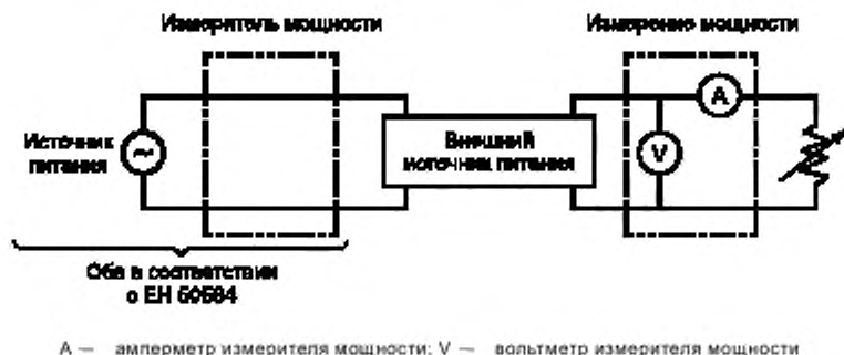
Рисунок 1 — Схема испытания
