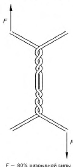
Рисунок 4 — Нагрузка на сетку для проверки прочности скрутки
