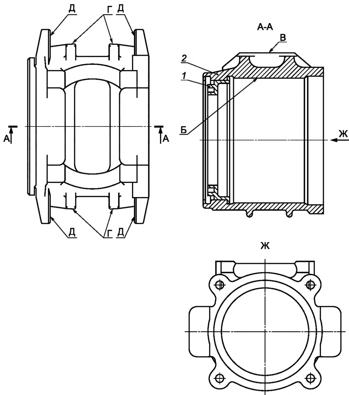
1 — лабиринтная часть; 2 — корпус бусы; Б — опорная поверхность под подшипник; В — опорная поверхность под боковую раму; Г — упорные стенки ограничителей продольных перемещений; Д — ограничители боковых перемещений; Ж — вид сбоку
