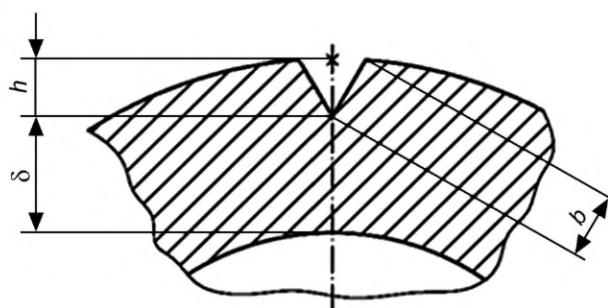
b — ширина обработанной фрезированием поверхности надреза; h — глубина надреза; \delta — остаточная толщина стенки
