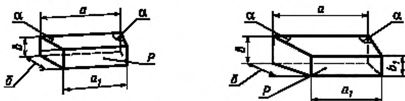
Рисунок 3 — Трапецидальный клин
