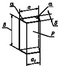
Рисунок 1 — Ребровый клин
