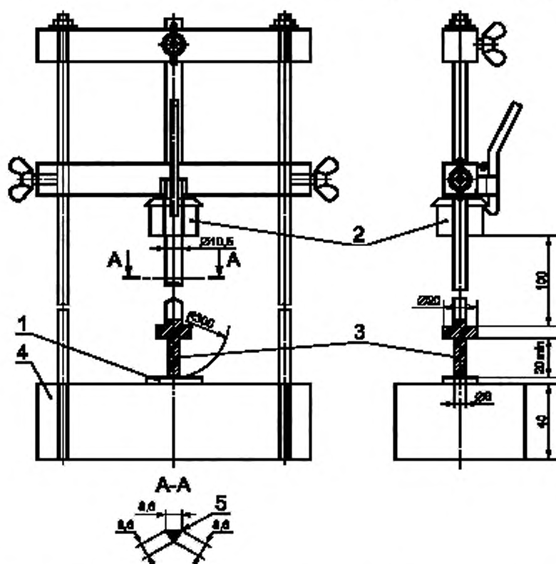
1 — образец; 2 — груз массой (100 \pm 1) г; 3 — промежуточная стальная вставка массой (100 \pm 1) г; 4 — стальная опора массой (10 \pm 1) кг; 5 — края закруглить
