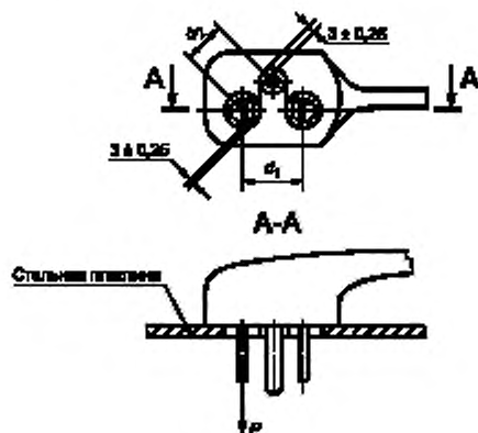
Рисунок 31 — Устройство для проверки механической прочности вилок
