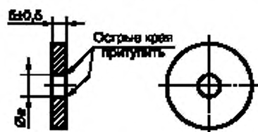
Непрямой калибр
