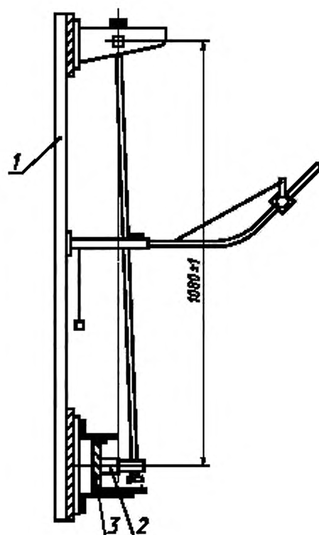
Рисунок 22 — Установка для проверки механической прочности соединителей
