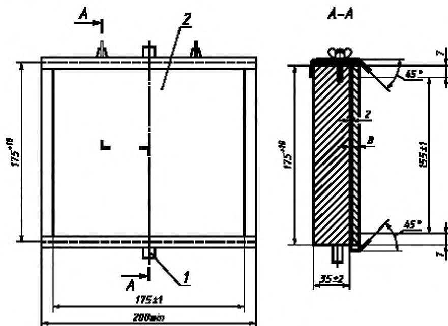
1 — ось вращения; 2 — фанерный лист; 3 — шарнир
