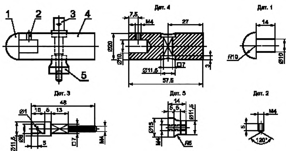
Рисунок 23 — Ударный элемент
