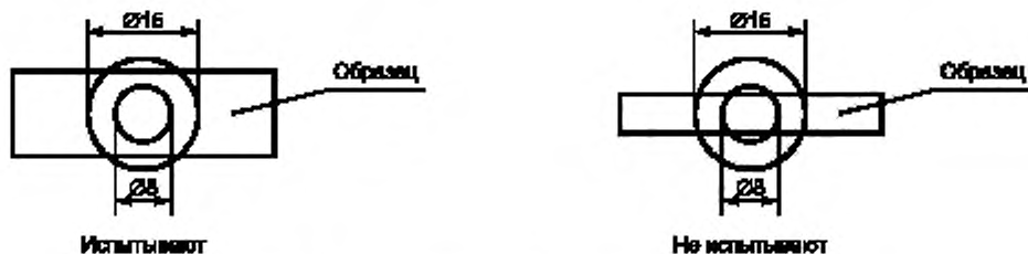
Рисунок 43 — Схематическое изображение требований 28.1.1
