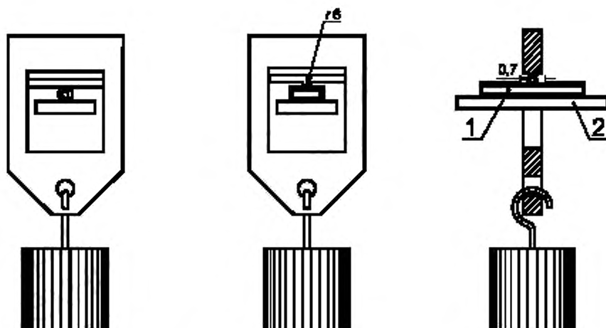
Вид спереди
