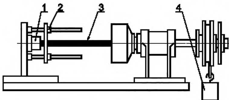
1 — испытуемый образец; 2 — зажимное приспособление; 3 — провод, шнур или кабель; 4 — груз
