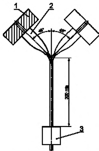
1 — устройство для закрепления образца; 2 — образец; 3 — груз
