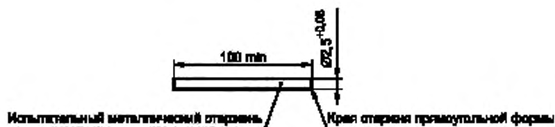
Рисунок 36 — Калибр для проверки пазов, отверстий и обратных конусов
