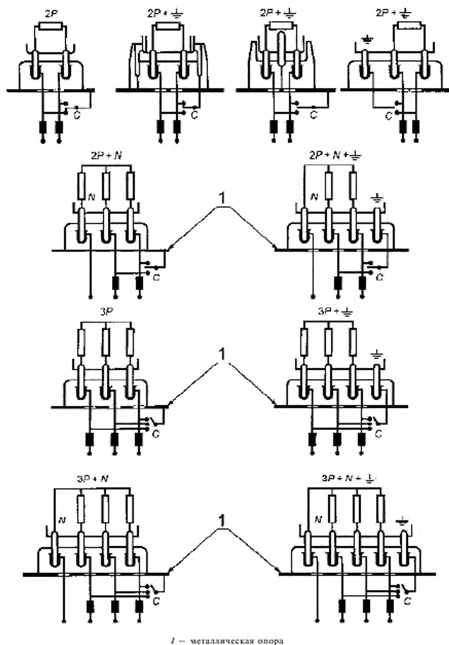
Рисунок 17 — Схемы соединения для испытания на нормальную работу
