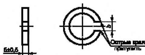
Непрямой калибр
