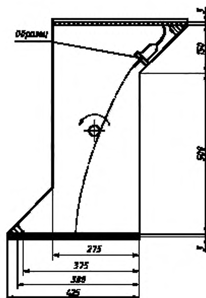
Рисунок 26 — Барабан для испытания соединителей на свободное падение
