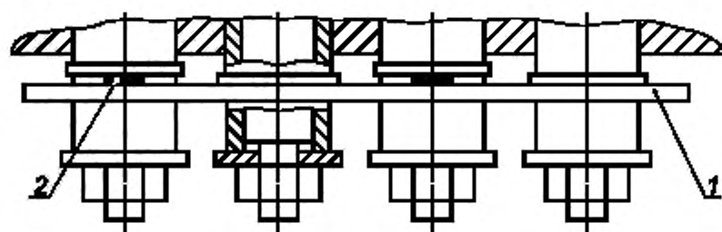
1 — поверочная линейка, 2 — щуп
