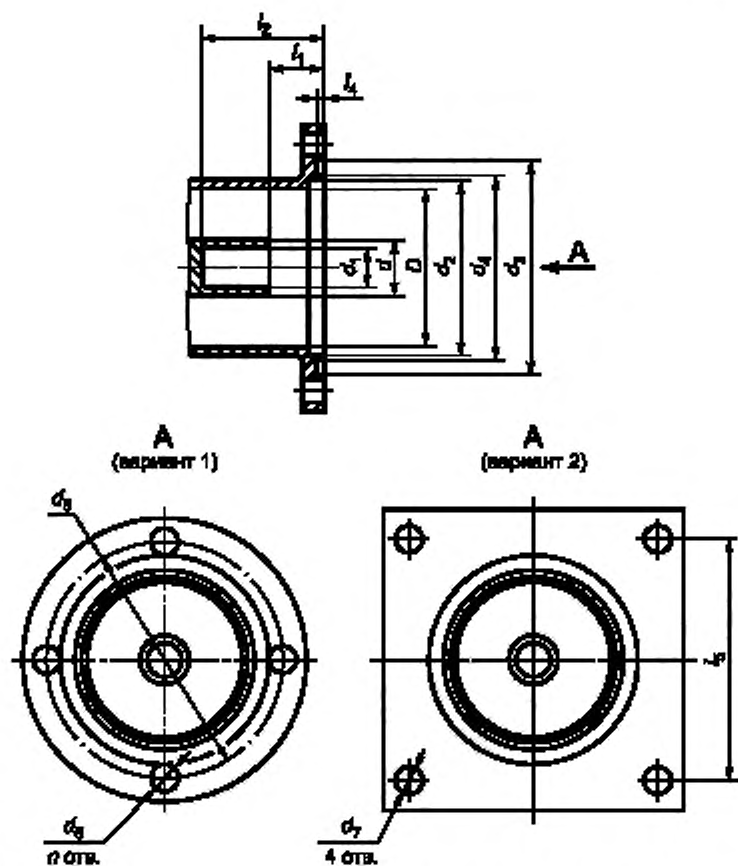
Рисунок А.2 — Присоединительные размеры СРМ фланцевого типа соединения
