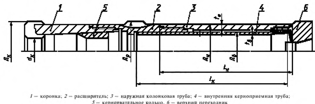
Рисунок 5 — Схема конструкции двойной колонковой трубы типа ТДК
