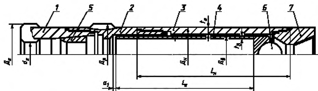
1 — коронка; 2 — расширитель; 3 — наружная колонковая труба; 4 — внутренняя керноприемная труба; 5 — кернорегулирующее кольцо; 6 — шаровая пята; 7 — верхний переходник
