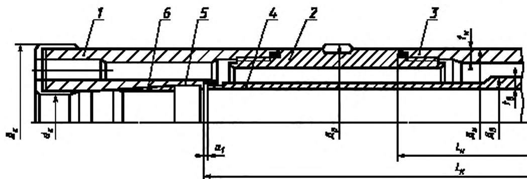
1 – коронка; 2 – расширитель; 3 – наружная колонковая труба; 4 – внутренняя керноприемная труба; 5 – корпус керноприемателя; 6 – кернорегулирующее кольцо
