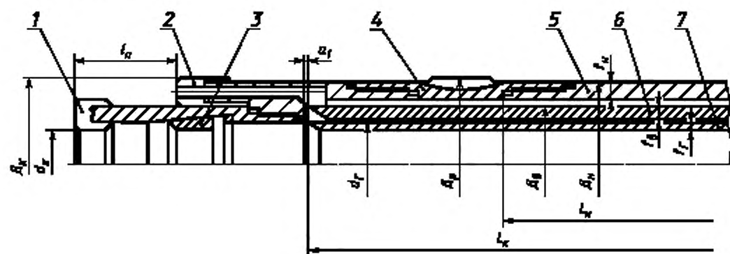
1 — пилот-коронка; 2 — формирующая коронка; 3 — керноразвальное кольцо; 4 — расширитель; 5 — наружная колонковая труба; 6 — внутренняя керноприемная труба; 7 — керноприемная гильза
