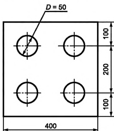
Рисунок 3 — Расположение анкеров на поверхности образца
