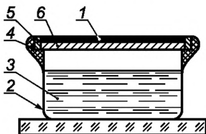
1 — испытуемый слой СФТК; 2 — стеклянная чашка; 3 — дистиллированная вода; 4 — герметизирующая мастика; 5 — слой парафина; 6 — основание (утеплитель)
