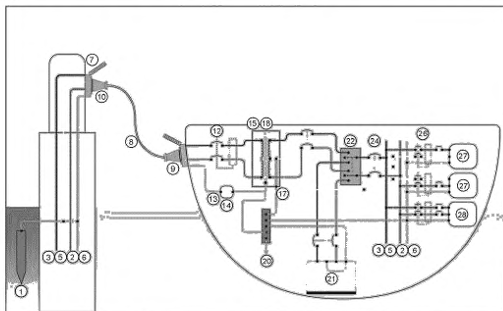
г) Система разделительного трансформатора с однофазным входом 240 В, выходом 120/240 В и генератором, демонстрирующая использование шины заземления основного переменного тока и УЗО/прерывателя берегового питания. Схема приведена с заземленным входом, подсоединенным к системе заземления судна (посредством дополнительного гальванического разъединителя) с преобразованием разъединительного трансформатора в трансформатор полярности.
