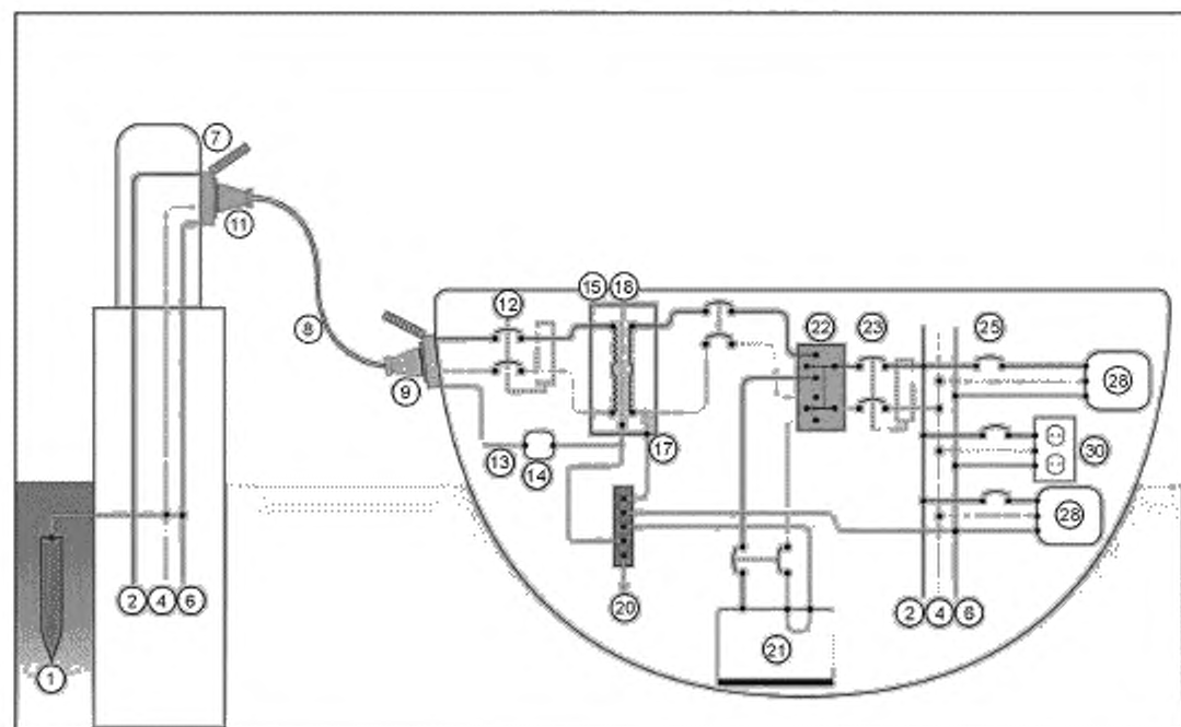
а) Система разделительного трансформатора с однофазным входом 230 В и выходом 230 В и генератора, демонстрирующая использование шины заземления основного переменного тока и УЗО/прерывателя берегового питания. Схема приведена с заземлением входа, подсоединенного к системе заземления судна (посредством дополнительного гальванического разъединителя) с преобразованием разделительного трансформатора в трансформатор полярности.
