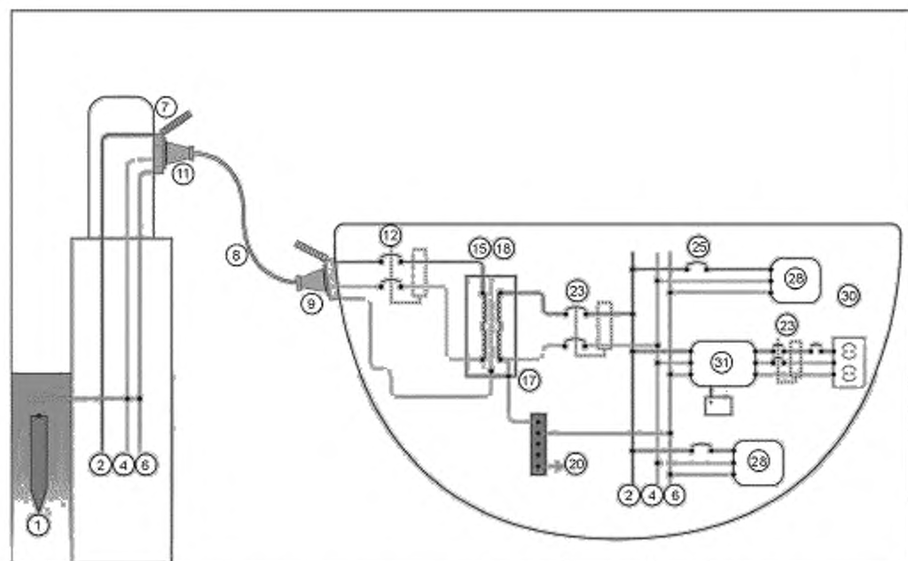
ф) Система разделительного трансформатора с однофазным входом/выходом 230 В и заземленной на судне вторичной обмоткой. Экран трансформатора, заземленный на берегу, показан с инвертером/зарядным устройством.
