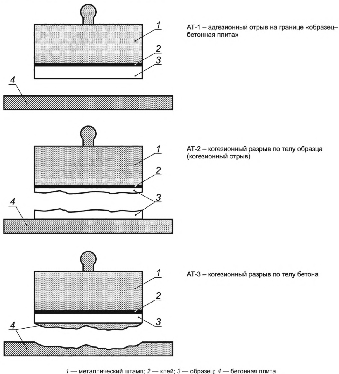
Рисунок 1 — Основные характерные виды отрыва образцов при определении прочности сцепления с бетонным основанием
