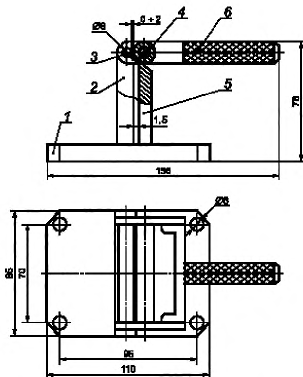
1 — плита; 2 — стойка; 3 — палец; 4 — ободья; 5 — упор; 6 — рукоятка
