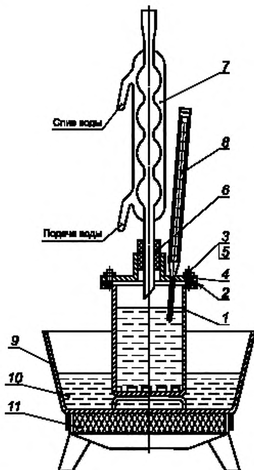
1 — стакан; 2 — прокладка резиновая; 3 — зажим; 4 — крышка; 5 — шпилька; 6 — резиновая пробка; 7 — шариковый холодильник; 8 — термометр; 9 — ванна; 10 — глицерин (вода); 11 — плитка
