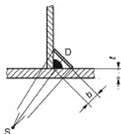
Рисунок 18 — Схема контроля при просвечивании угловых сварных швов
