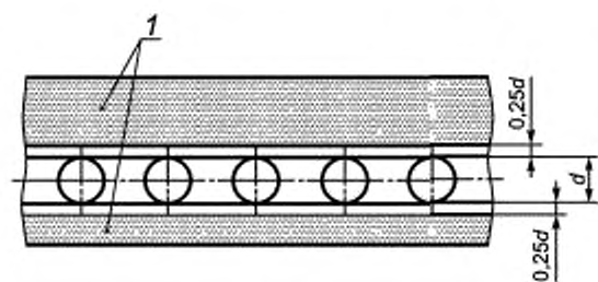
1 — обкладки
