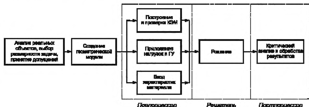
Рисунок 1 — Алгоритм проведения КМ НДС
