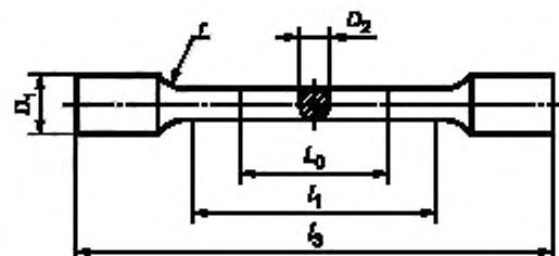
Рисунок В.3 — Образец для испытания типа 4
