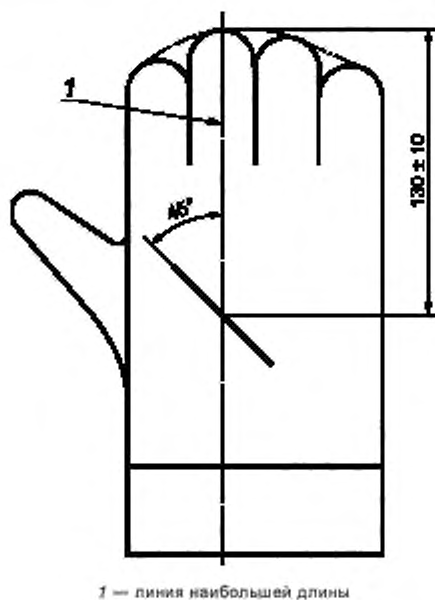
Рисунок 8 — Позиция 4: необязательный надрез вдоль тыльной стороны перчатки на правую руку конструкции В
