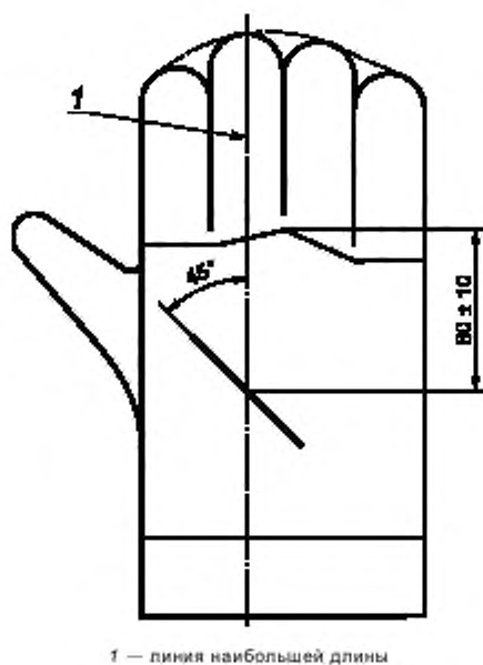
Рисунок 7 — Позиция 4: необязательный надрез вдоль тыльной стороны перчатки на правую руку
